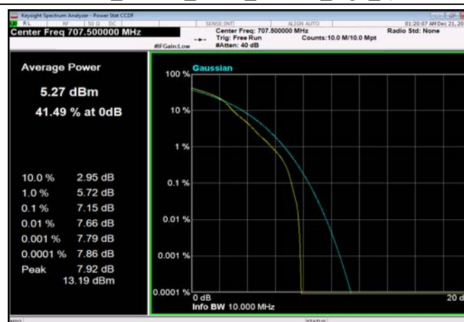
FDD12_10MHz_707.5_OneRB_high_Q16
