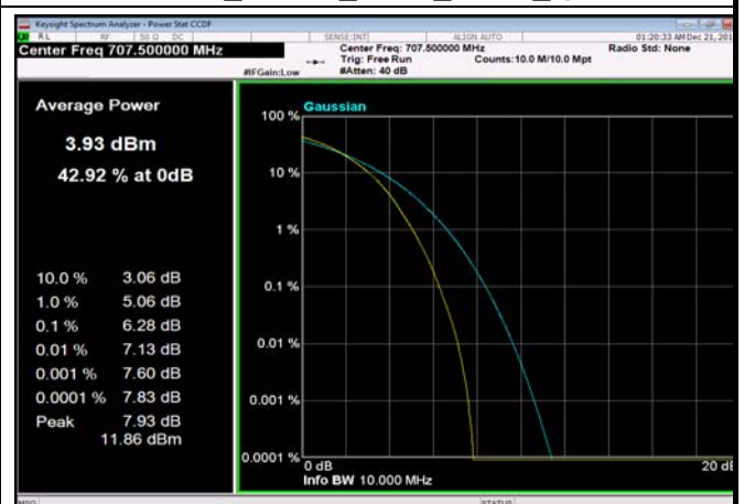
FDD12_10MHz_707.5_fullRB_Q16
