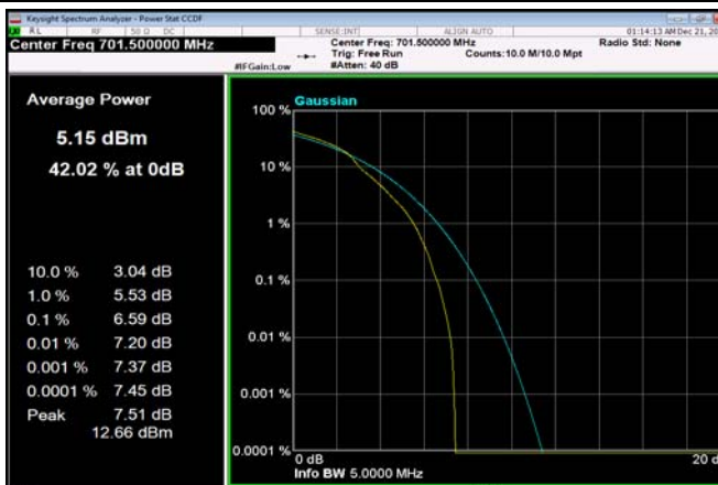
FDD12_5MHz_701.5_OneRB_high_Q16
