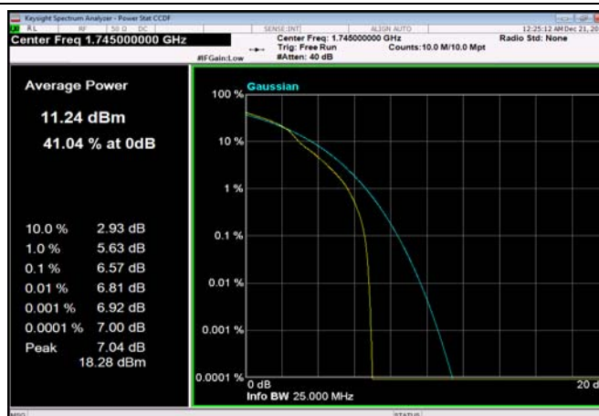
FDD04_20MHz_1745_OneRB_high_Q16
