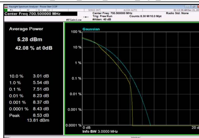
FDD12_3MHz_700.5_OneRB_high_Q16
