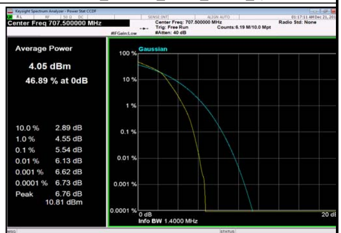
FDD12_1.4MHz_707.5_fullRB_Q16
