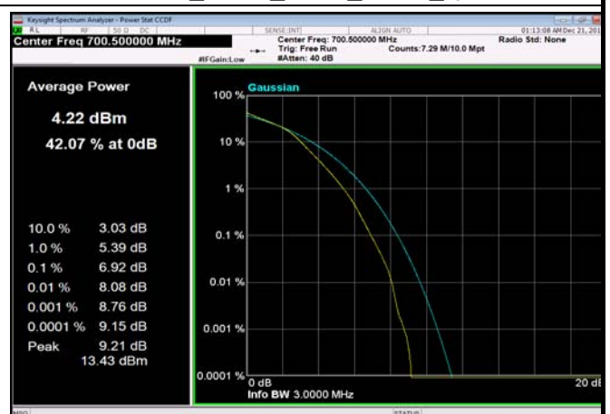
FDD12_3MHz_700.5_fullRB_Q16
