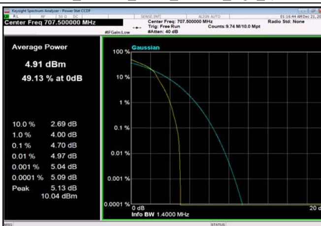
FDD12_1.4MHz_707.5_OneRB_high_Q16
