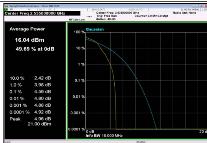
FDD07_15MHz_2535_OneRB_high_Q16
