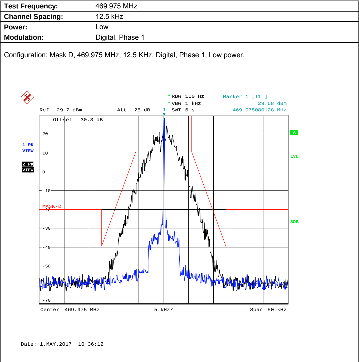
Plot 5.8.4.2.12. Emission Mask D, Low Power
