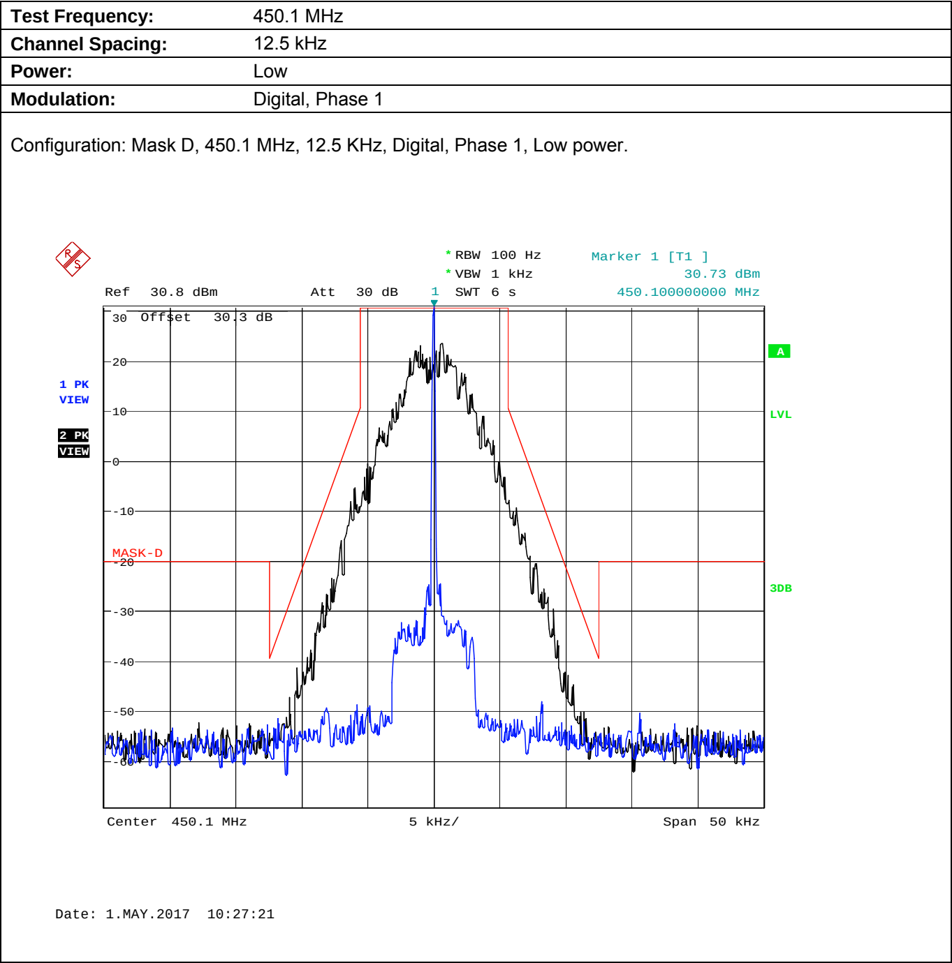
Plot 5.8.4.2.11. Emission Mask D, Low Power
