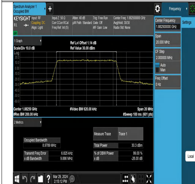
Band25-10MHz-QPSK-26365-50RB#0-PASS
