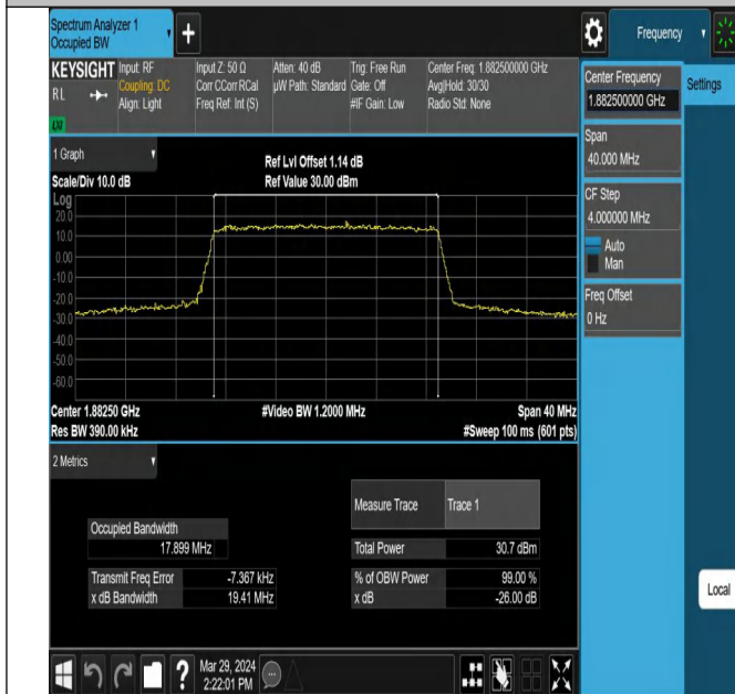
Band25-20MHz-QPSK-26365-100RB#0-PASS
