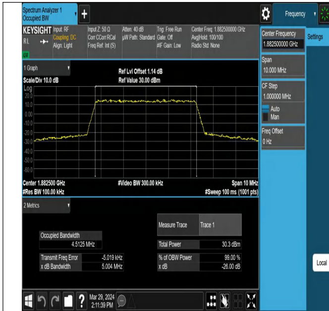
Band25-5MHz-QPSK-26365-25RB#0-PASS
