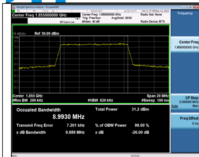
Band2-10MHz-QPSK-18650-50RB#0-PASS
