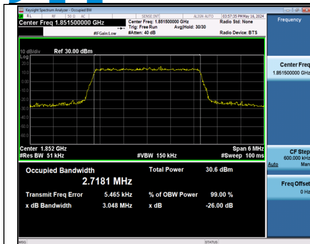
Band2-3MHz-QPSK-18615-15RB#0-PASS
