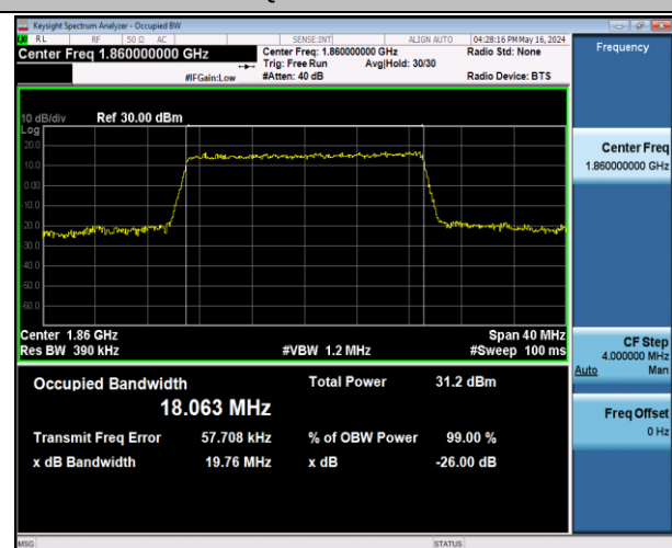
Band2-20MHz-16QAM-18700-100RB#0-PASS
