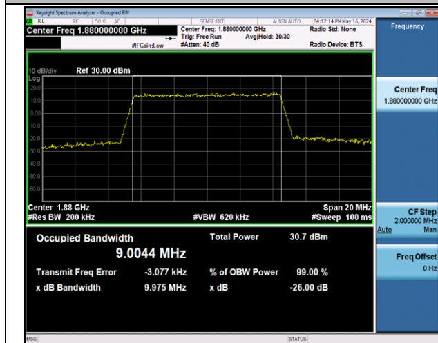
Band2-10MHz-16QAM-18900-50RB#0-PASS
