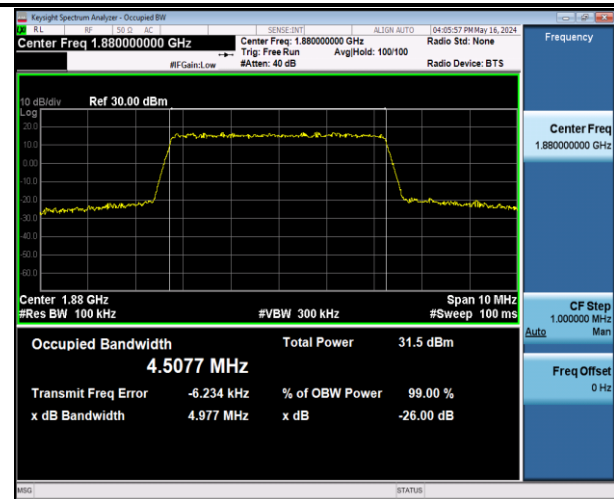
Band2-5MHz-QPSK-18900-25RB#0-PASS
