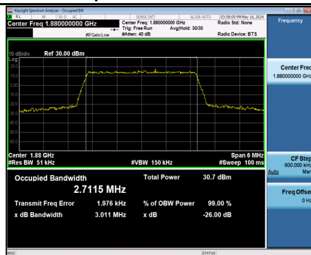
Band2-3MHz-QPSK-18900-15RB#0-PASS
