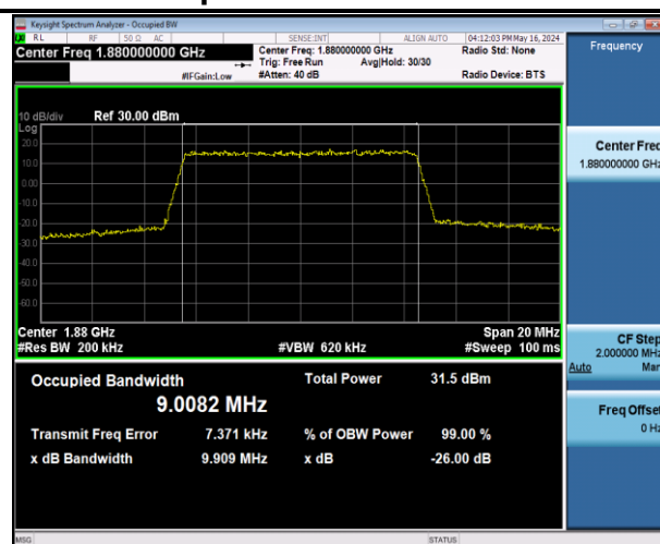
Band2-10MHz-QPSK-18900-50RB#0-PASS
