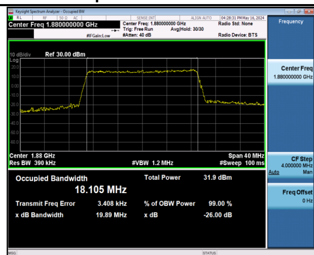
Band2-20MHz-QPSK-18900-100RB#0-PASS
