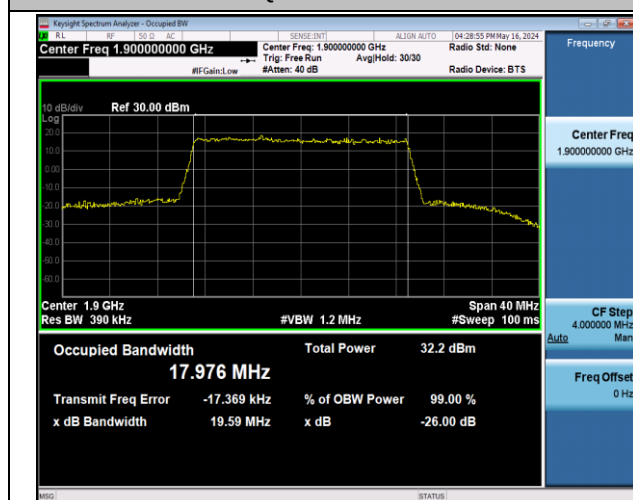
Band2-20MHz-QPSK-19100-100RB#0-PASS
