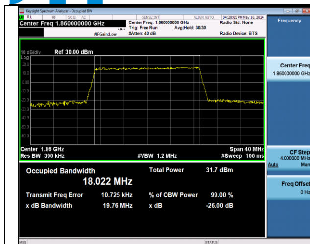
Band2-20MHz-QPSK-18700-100RB#0-PASS
