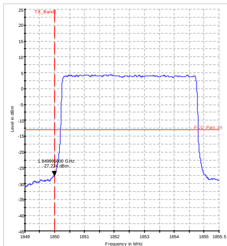
Diagram 37.206a_ch18625_25RB_low_QPSK
