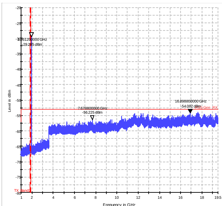
Diagram 50_01_CH_18900_QPSK_RB_Full_FDD2
