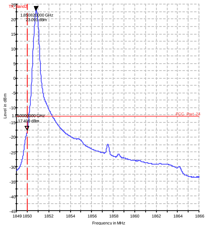
Diagram 37.209b_ch18675_1RB_low_QAM
