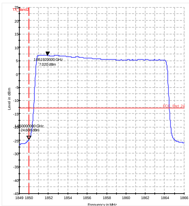
Diagram 37.210a_ch18675_75RB_low_QPSK
