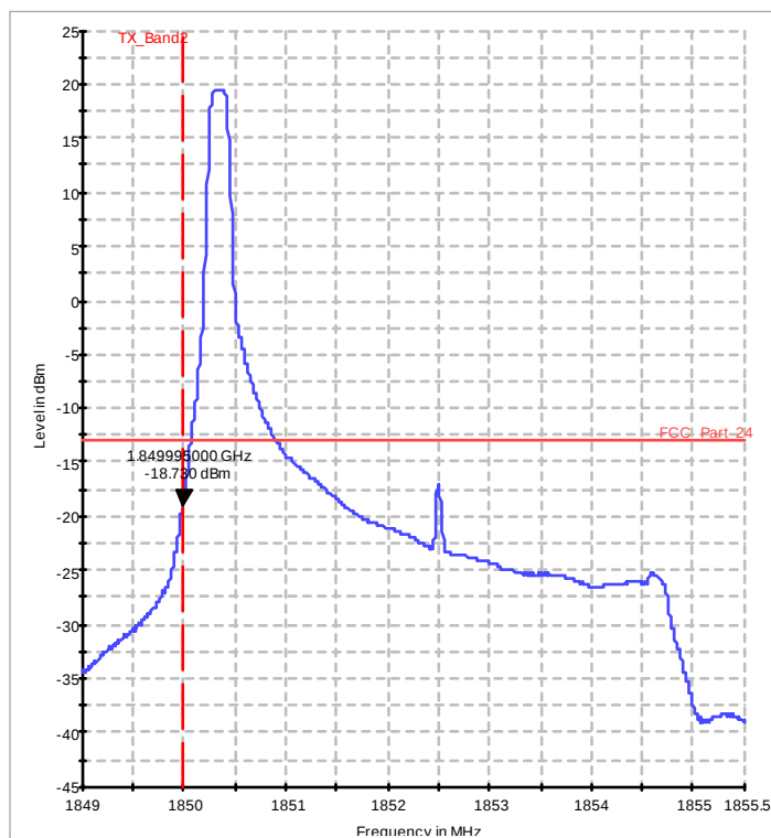
Diagram 37.205a_ch18625_1RB_low_QPSK
