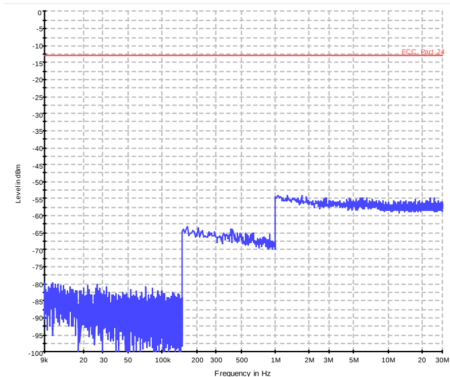
Diagram 36.22a_CSE_Ch18900_BW_15_1RB_low_QPSK_Sweep1
