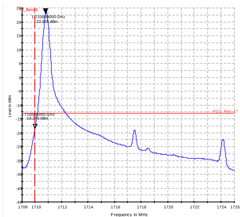
Diagram 37.409a_Ch20025_BW_15_1RB_low_QPSK
