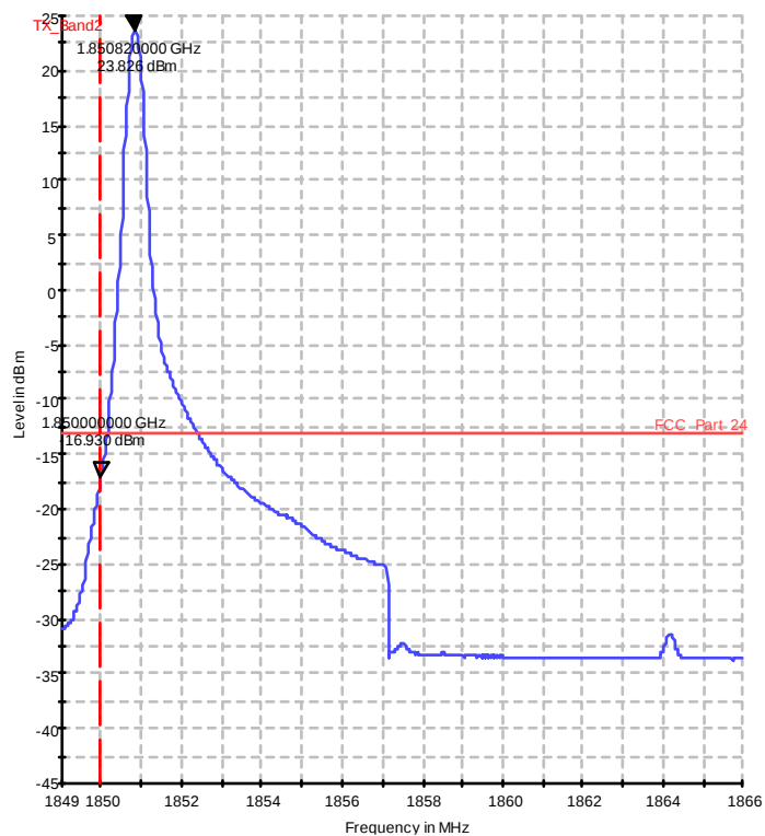
Diagram 37.209a_ch18675_1RB_low_QPSK
