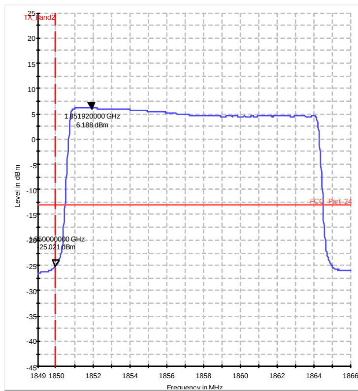
Diagram 37.210b_ch18675_75RB_low_QAM
