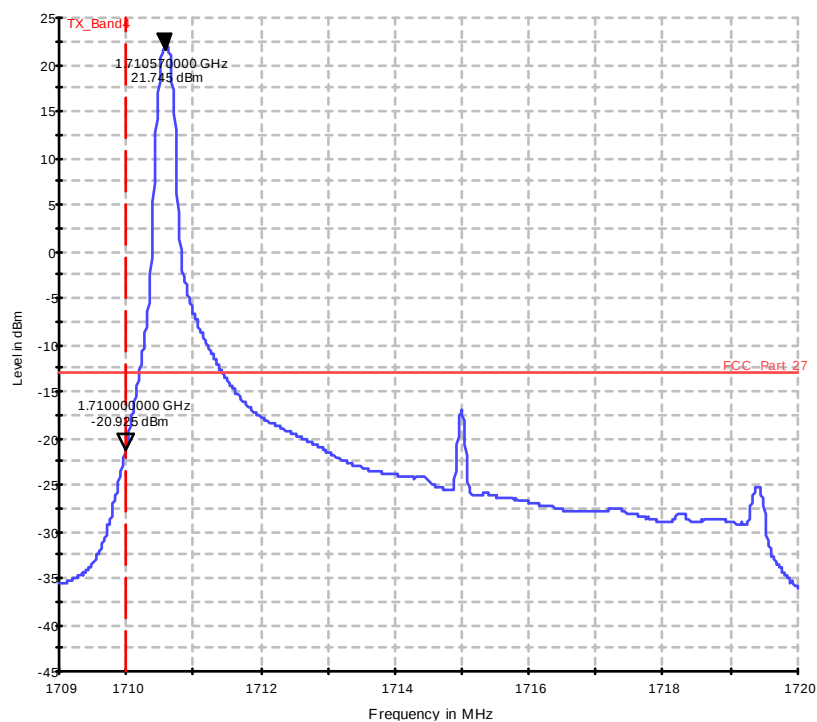
Diagram 37.407a_Ch20000_BW_10_1RB_low_QPSK
