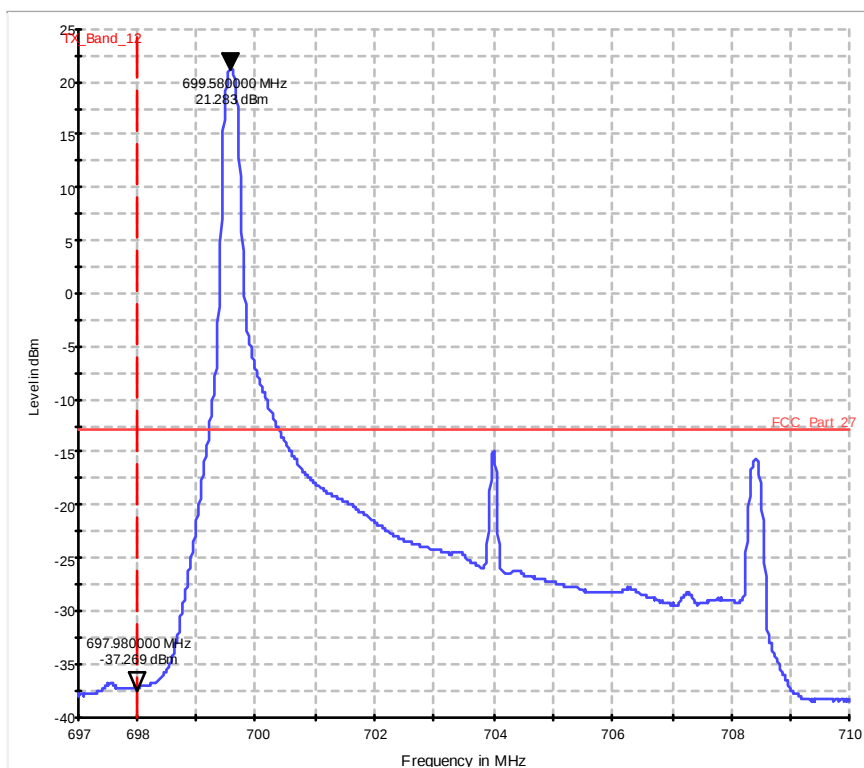
Diagram 37.1207a_Ch23060_BW_10_1RB_low_QPSK
