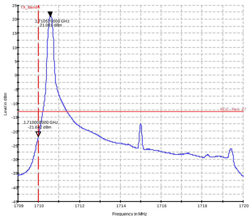
Diagram 37.407b_Ch20000_BW_10_1RB_low_16QAM
