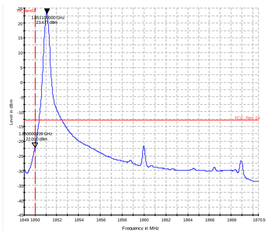
Diagram 37.211a_ch18700_1RB_low_QPSK
