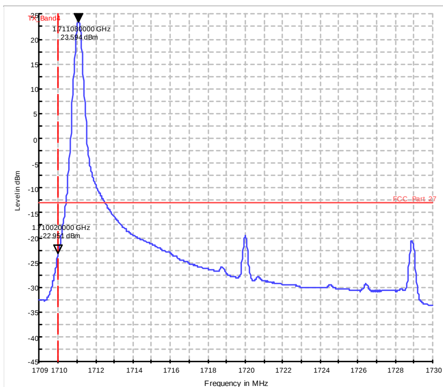
Diagram 37.411a_Ch20050_BW_20_1RB_low_QPSK
