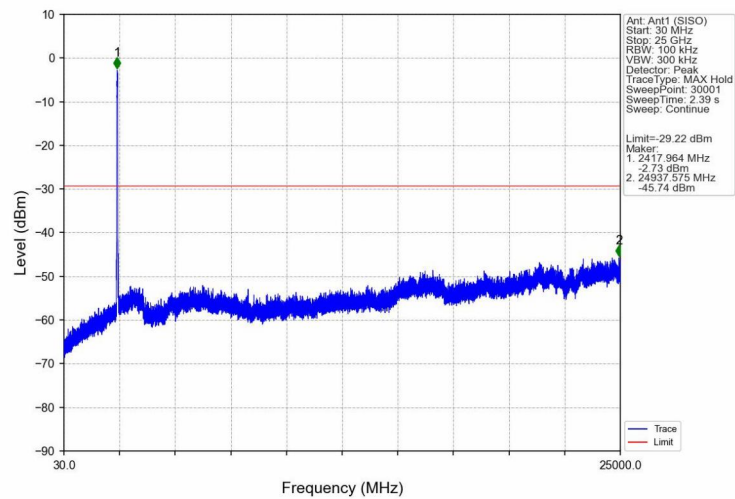
802.11n(HT40)_MCH_2437MHz_Ant1 (SISO)_NTNV
