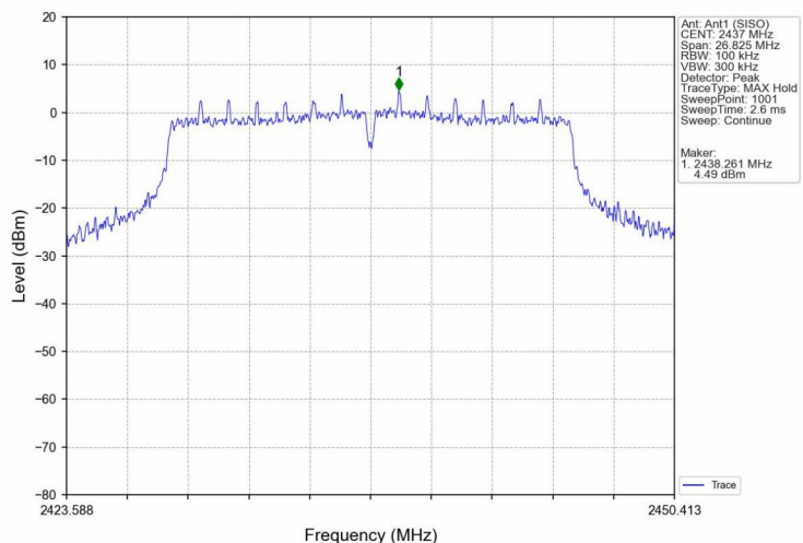
802.11n(HT20)_MCH_2437MHz_Ant1 (SISO)_NTNV
