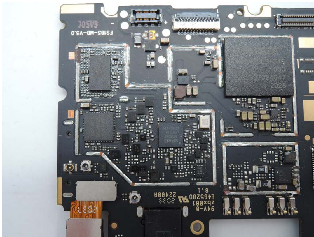
IC Details 3
