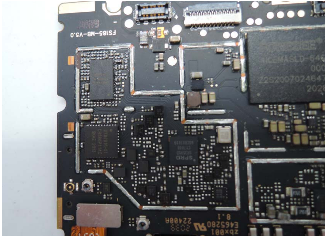
IC Details 4
