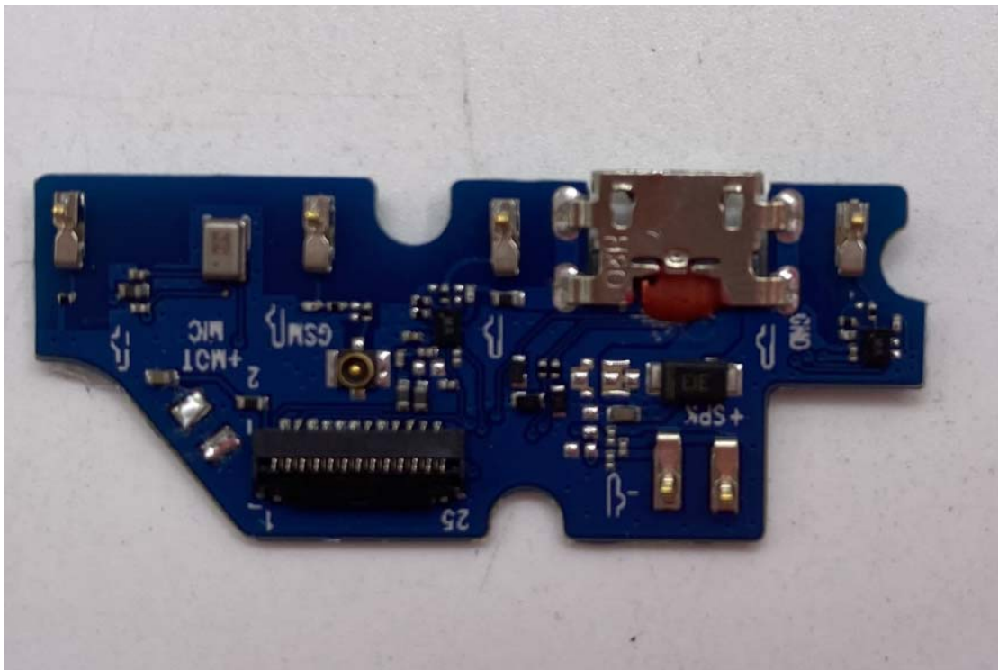
IC Details 7
