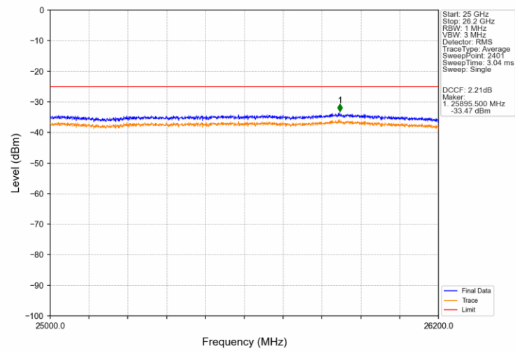
Band38_20MHz_QPSK_MCH_2595MHz_RB_1_0_NTNV
