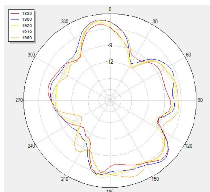
V Phi=90
