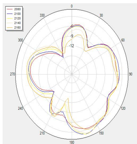
V Phi=90
