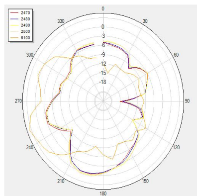
H Theta=90
