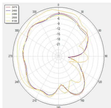
V Phi=90
