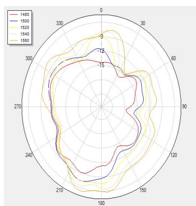
V Phi=90
