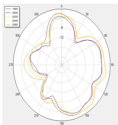
V Phi=90
