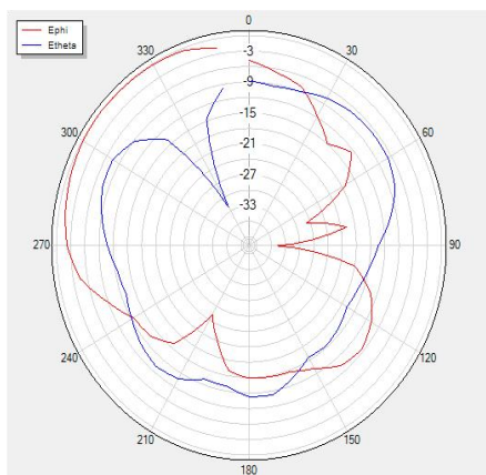
H Theta=90 freq=2580MHz
