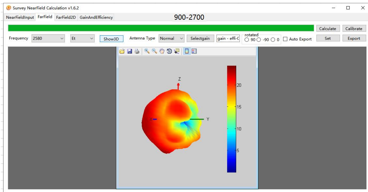
H Theta=90 freq=2580MHz
