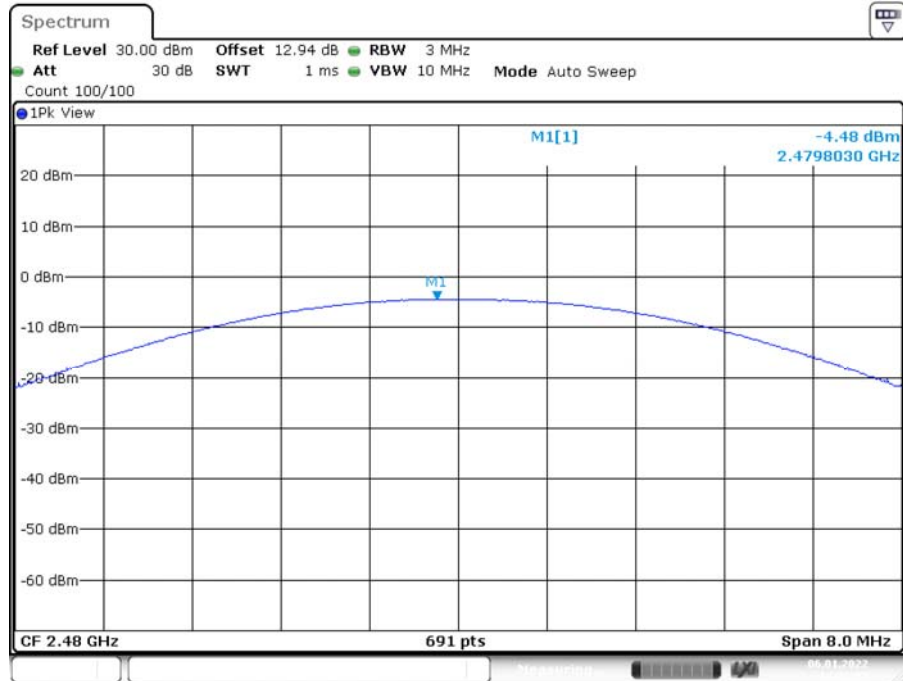
DH1_Ant1_2480
