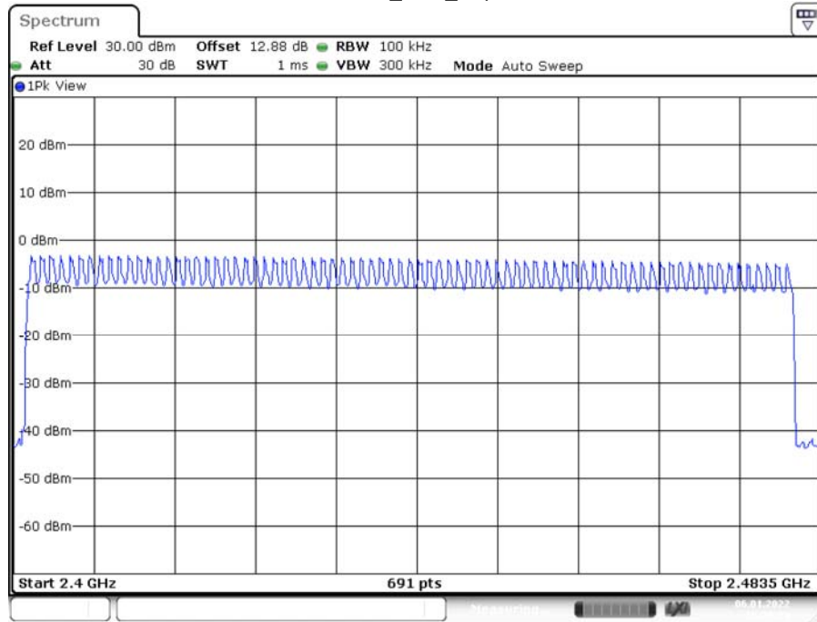
2DH1_Ant1_Hop
