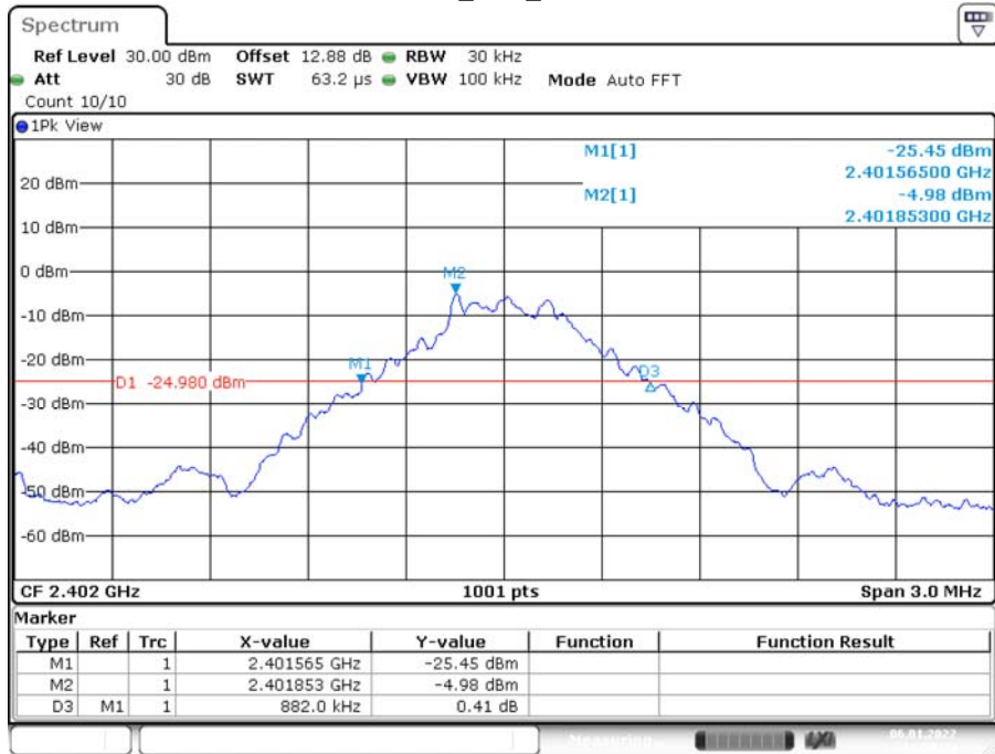
DH1_Ant1_2402
