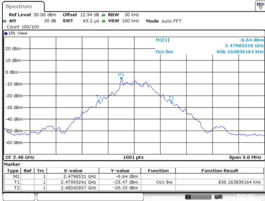
DH1_Ant1_2480
