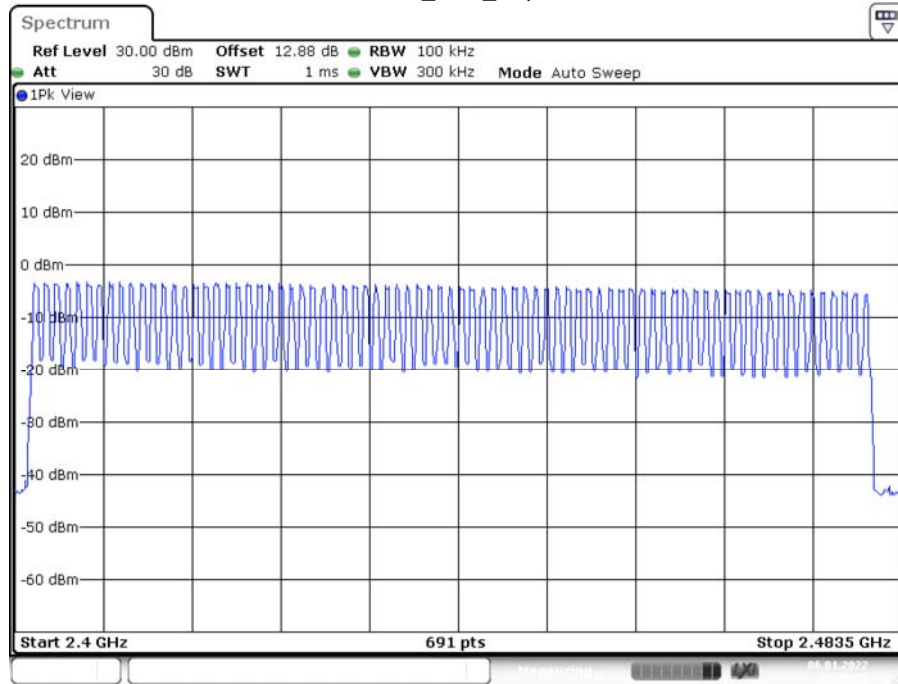
DH1_Ant1_Hop
