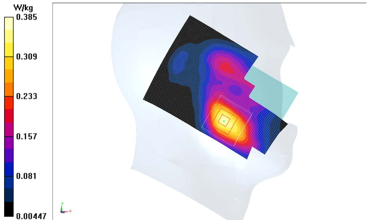
Fig.11 LTE Band4
