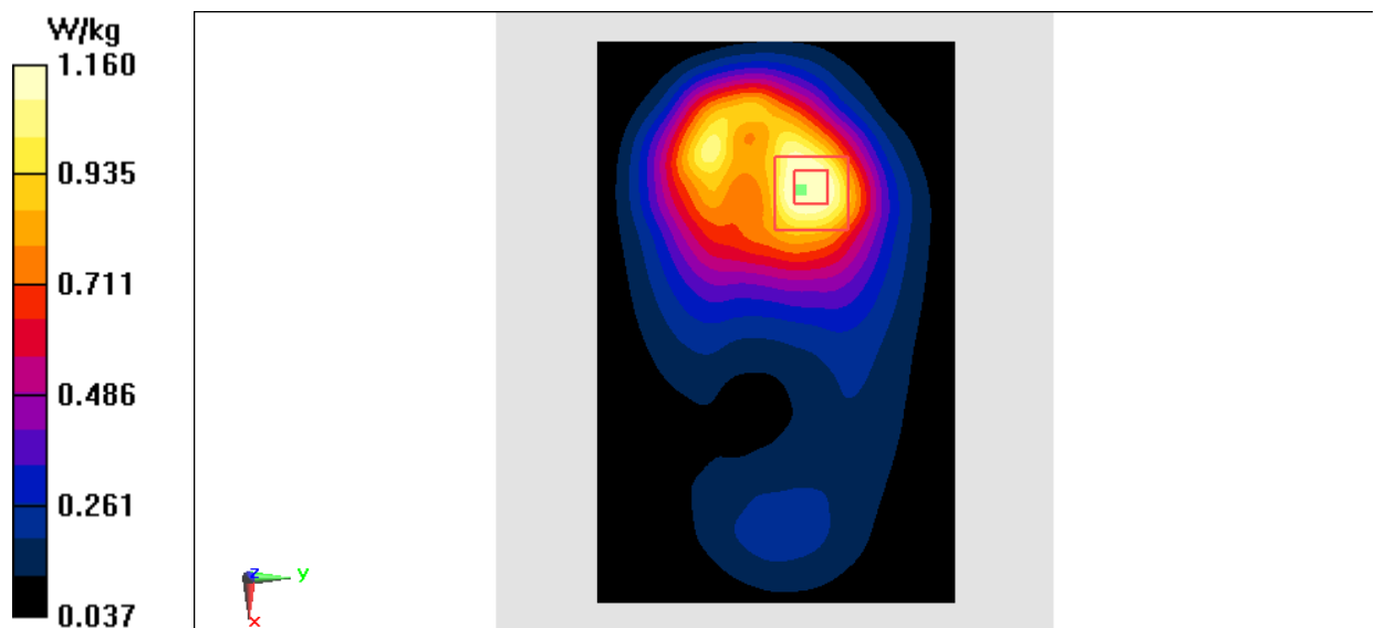
Fig.12 LTE Band4
