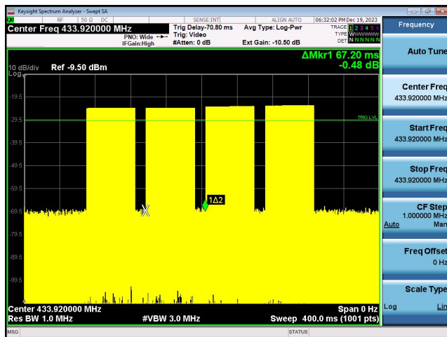
433.92 MHz: Burst 1
