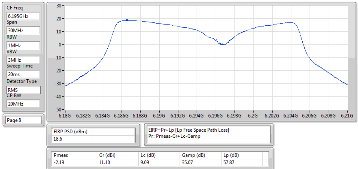
EIRP PSD;Band:6.2G;ax20;BWch:20MHz;Nss:1,(M0);Nant:4;Ch:6195MHz;TX
