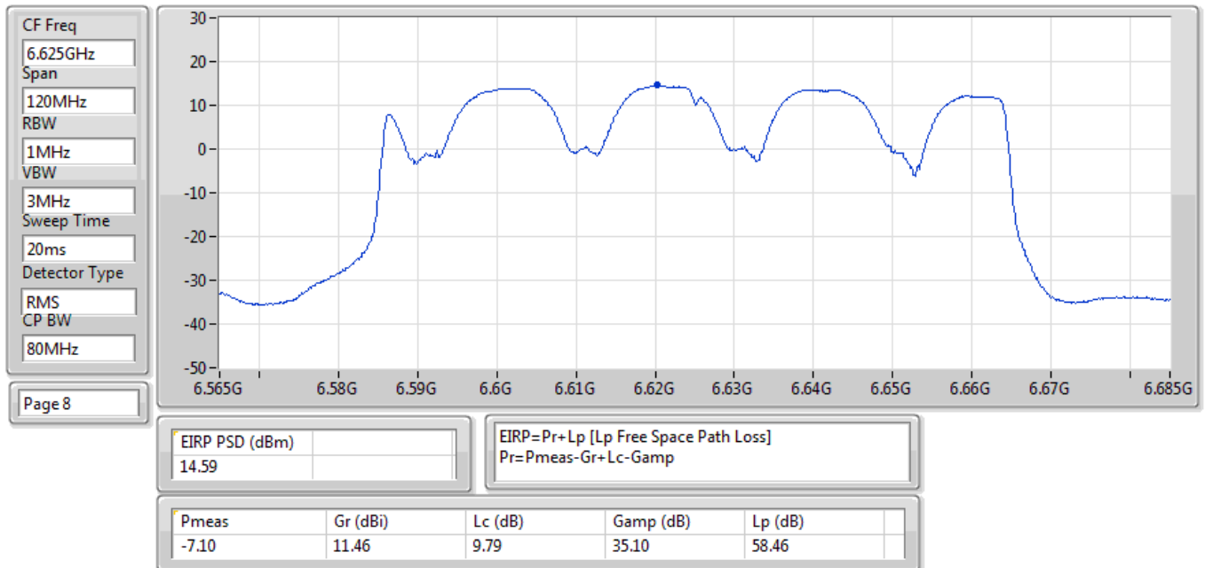
EIRP PSD;Band:6.7G;ax80;BWch:80MHz;Nss:1,(M0);Nant:4;Ch:6625MHz;TX
