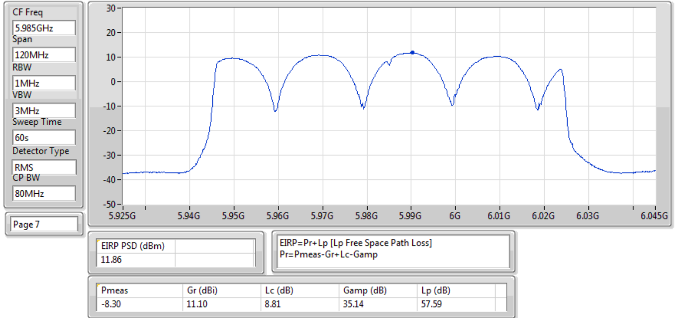
EIRP PSD;Band:6.2G;ax80;BWch:80MHz;Nss:1,(M0);Nant:4;Ch:5985MHz;TX
