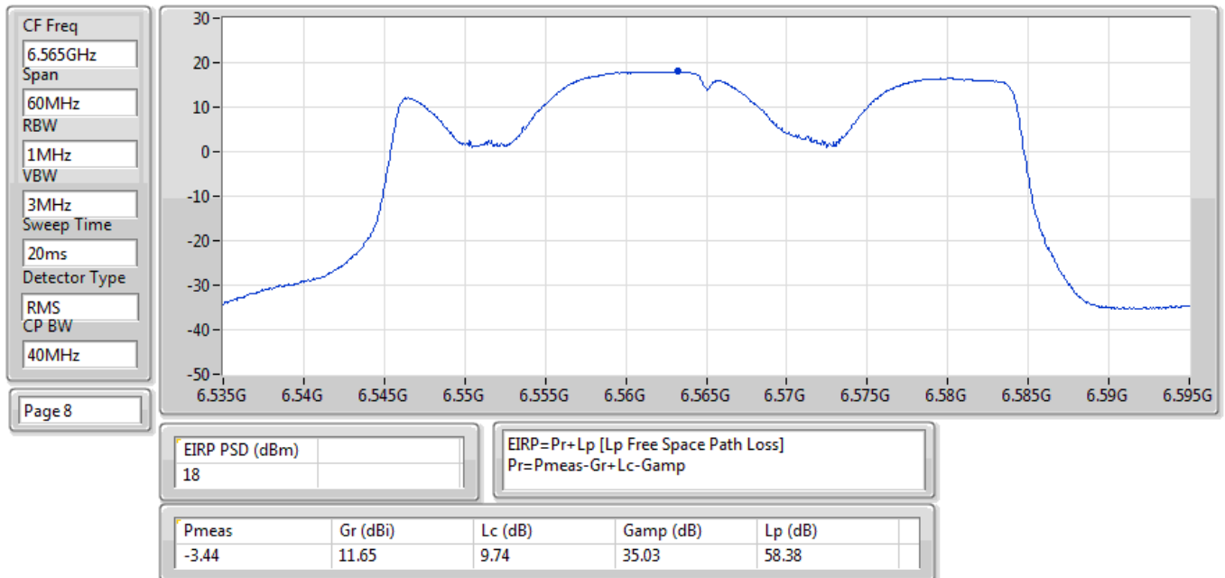
EIRP PSD;Band:6.7G;ax40;BWch:40MHz;Nss:1,(M0);Nant:4;Ch:6565MHz;TX
