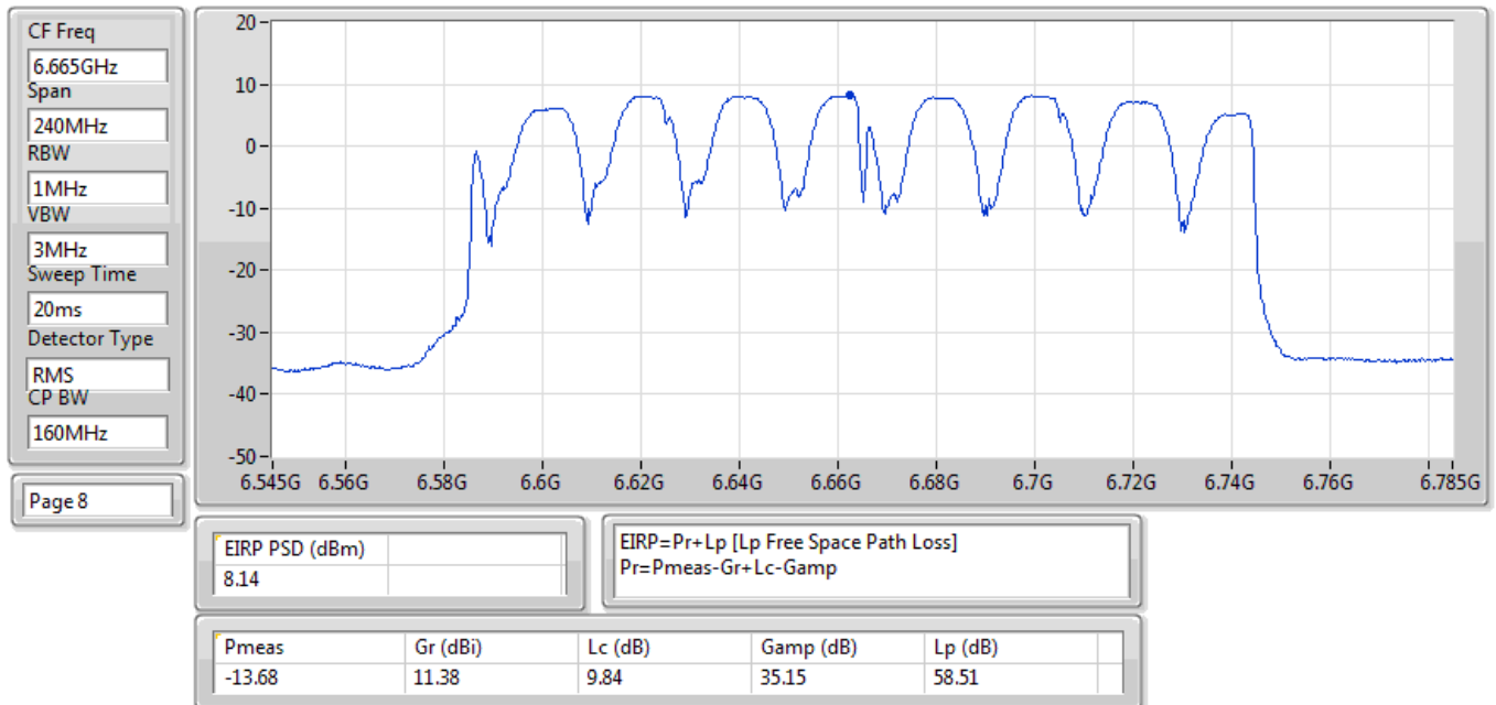
EIRP PSD;Band:6.7G;ax160;BWch:160MHz;Nss:1,(M0);Nant:4;Ch:6665MHz;TX
