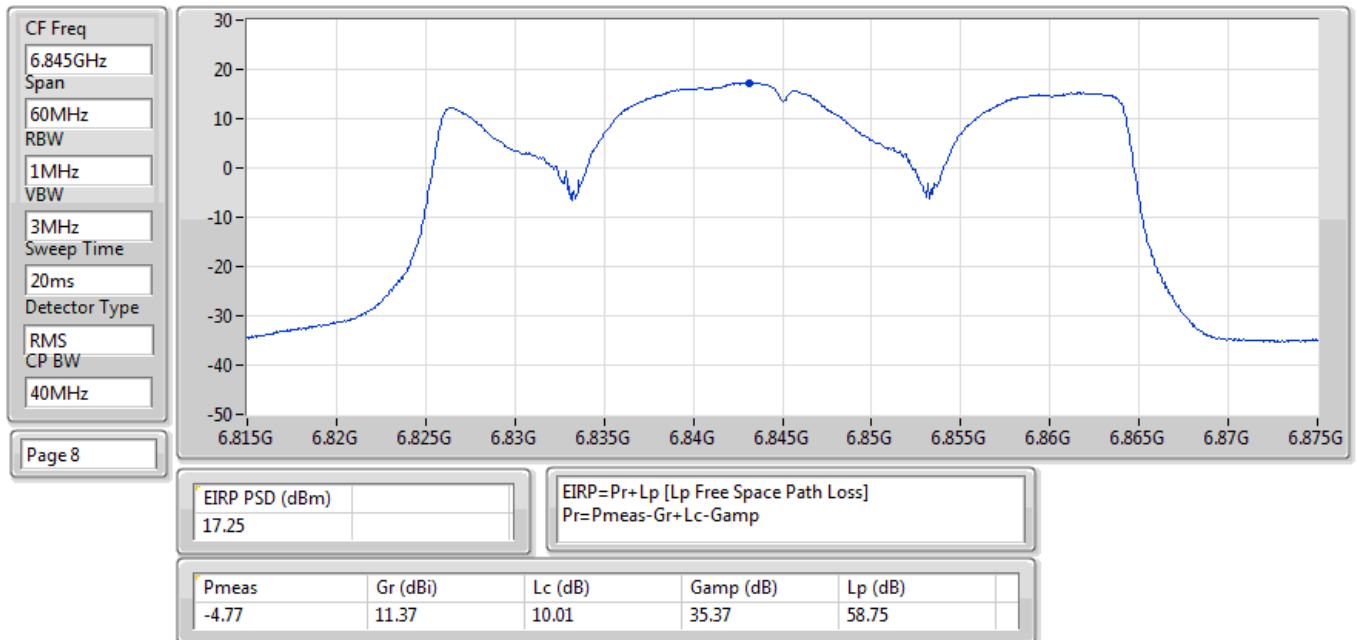
EIRP PSD;Band:6.7G;ax40;BWch:40MHz;Nss:1,(M0);Nant:4;Ch:6845MHz;TX
