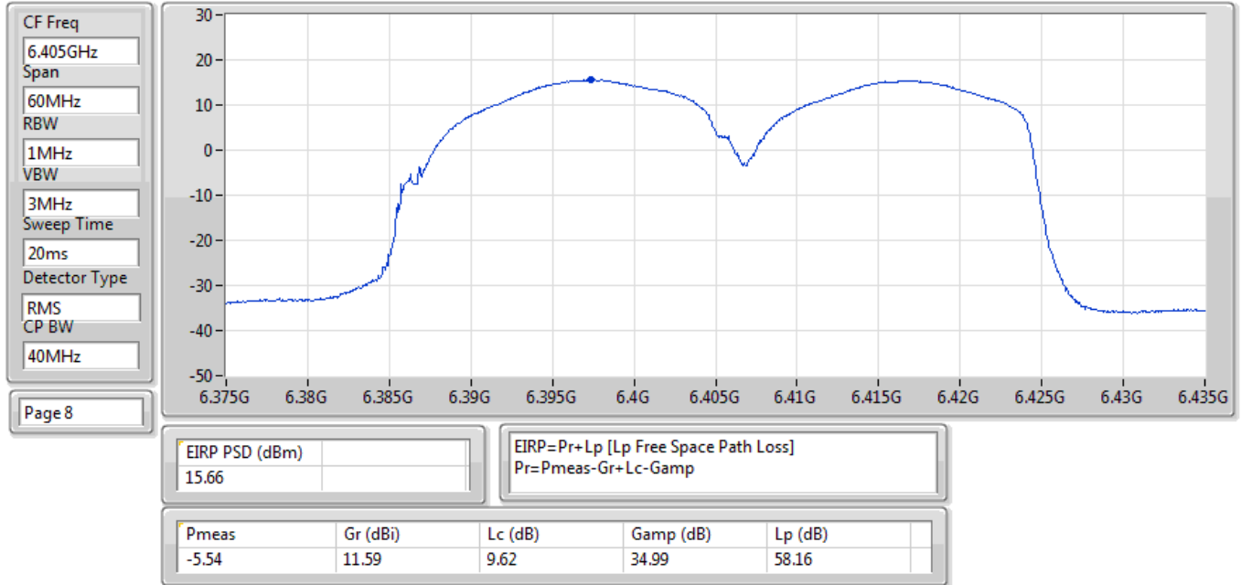
EIRP PSD;Band:6.2G;ax40;BWch:40MHz;Nss:1,(M0);Nant:4;Ch:6405MHz;TX
