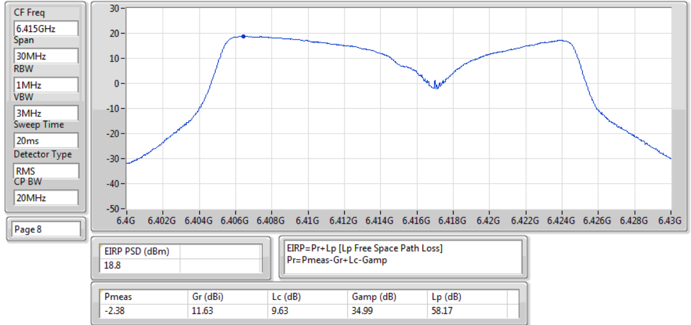
EIRP PSD;Band:6.2G;ax20;BWch:20MHz;Nss:1,(M0);Nant:4;Ch:6415MHz;TX
