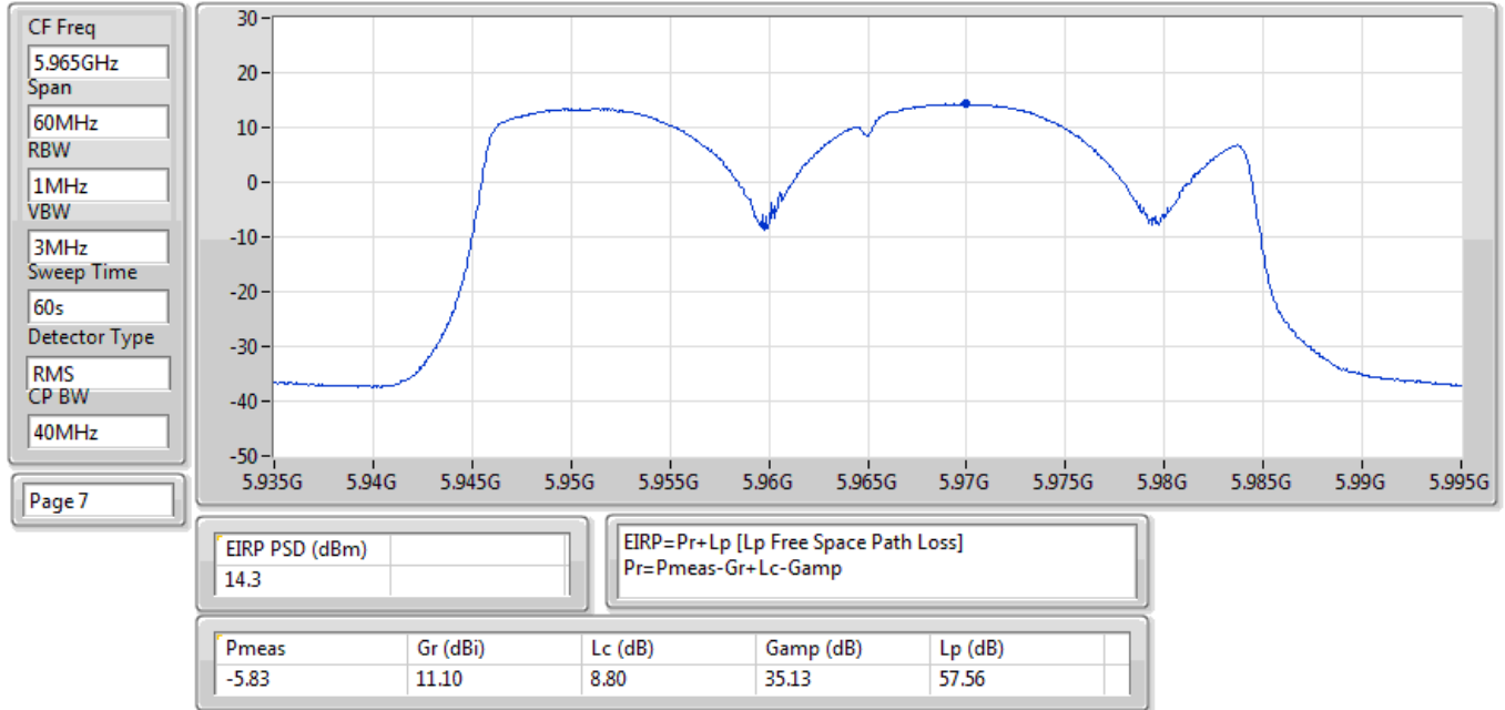
EIRP PSD;Band:6.2G;ax40;BWch:40MHz;Nss:1,(M0);Nant:4;Ch:5965MHz;TX
