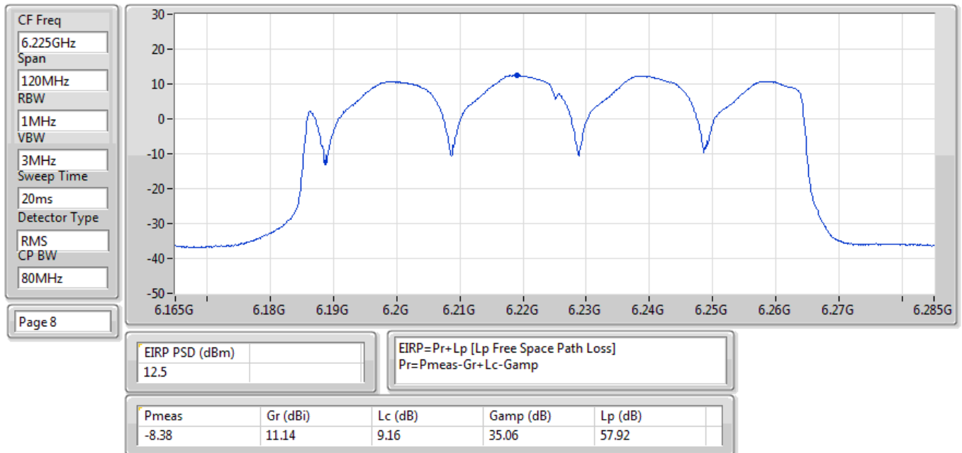
EIRP PSD;Band:6.2G;ax80;BWch:80MHz;Nss:1,(M0);Nant:4;Ch:6225MHz;TX
