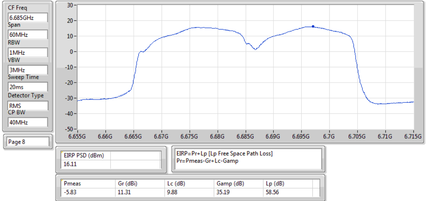
EIRP PSD;Band:6.7G;ax40;BWch:40MHz;Nss:1,(M0);Nant:4;Ch:6685MHz;TX
