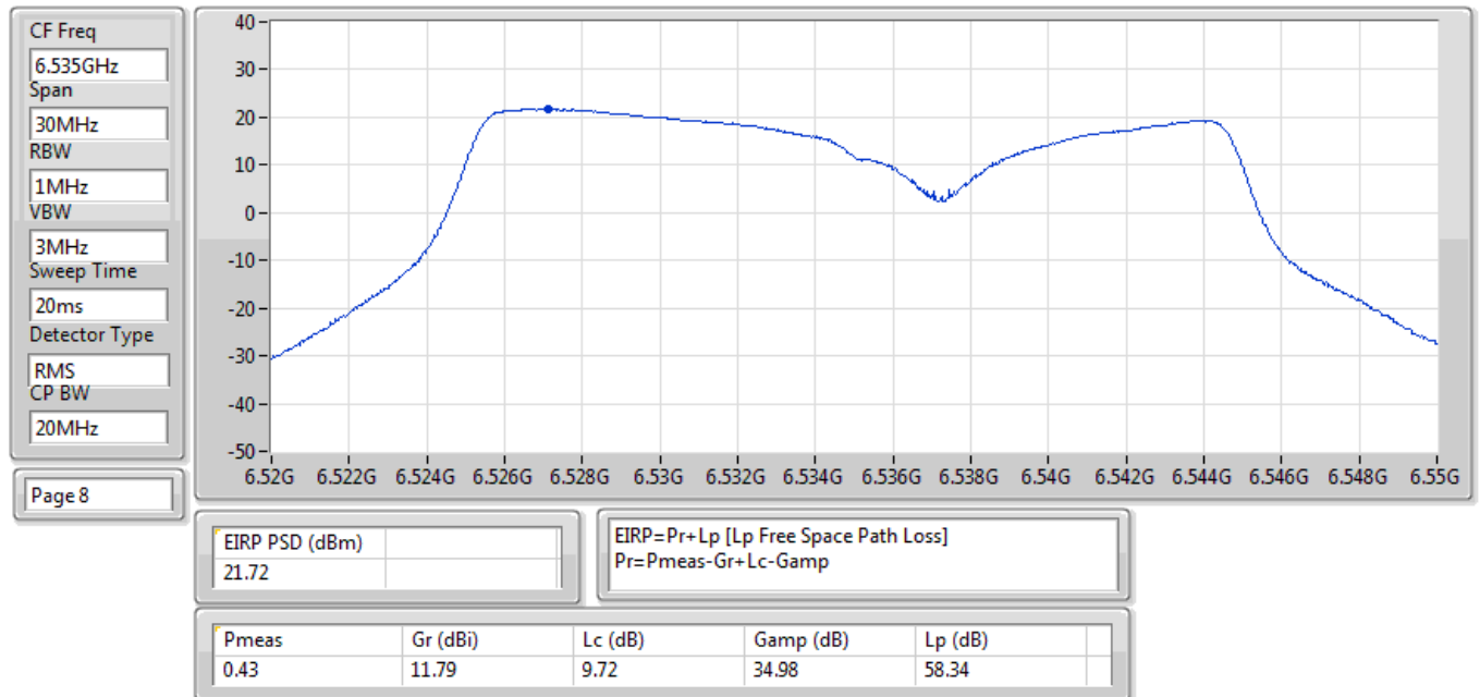
EIRP PSD;Band:6.7G;ax20;BWch:20MHz;Nss:1,(M0);Nant:4;Ch:6535MHz;TX
