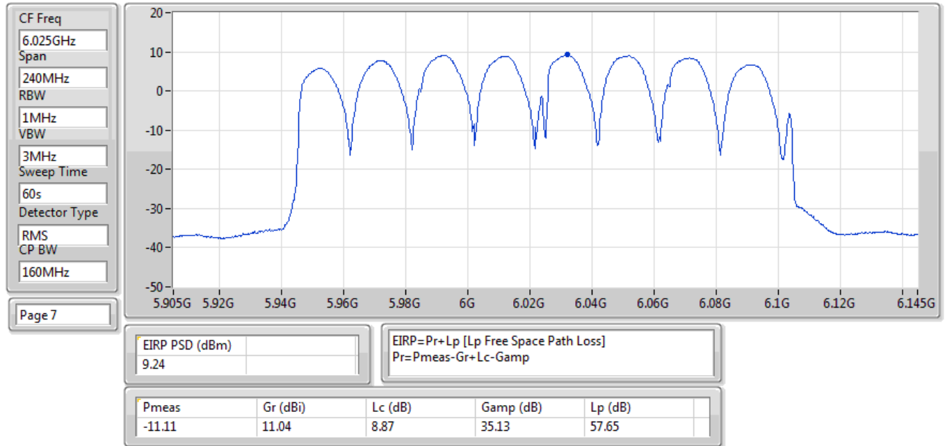
EIRP PSD;Band:6.2G;ax160;BWch:160MHz;Nss:1;(M0);Nant:4;Ch:6025MHz;TX
