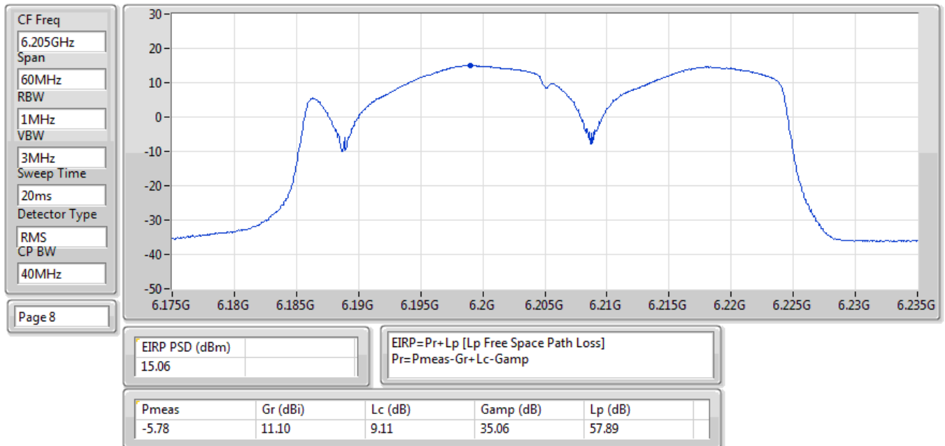
EIRP PSD;Band:6.2G;ax40;BWch:40MHz;Nss:1,(M0);Nant:4;Ch:6205MHz;TX
