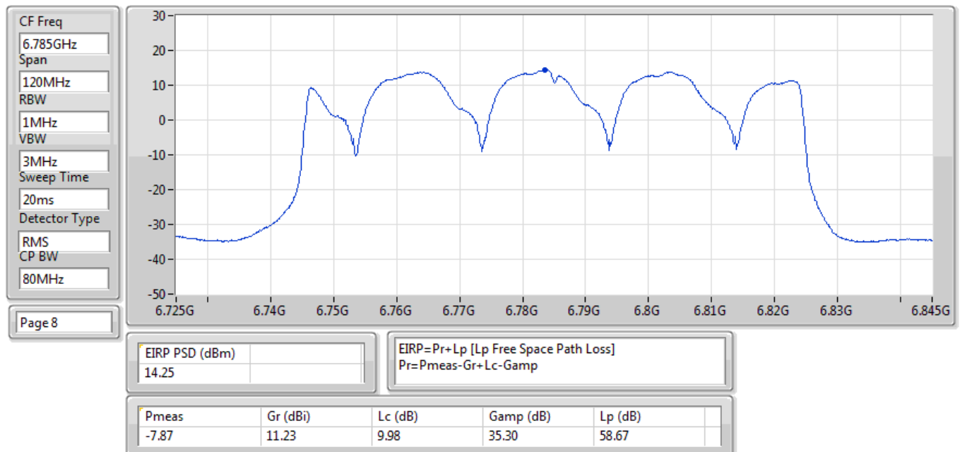
EIRP PSD;Band:6.7G;ax80;BWch:80MHz;Nss:1,(M0);Nant:4;Ch:6785MHz;TX
