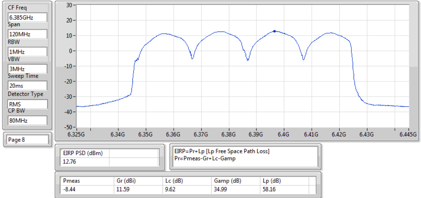
EIRP PSD;Band:6.2G;ax80;BWch:80MHz;Nss:1,(M0);Nant:4;Ch:6385MHz;TX
