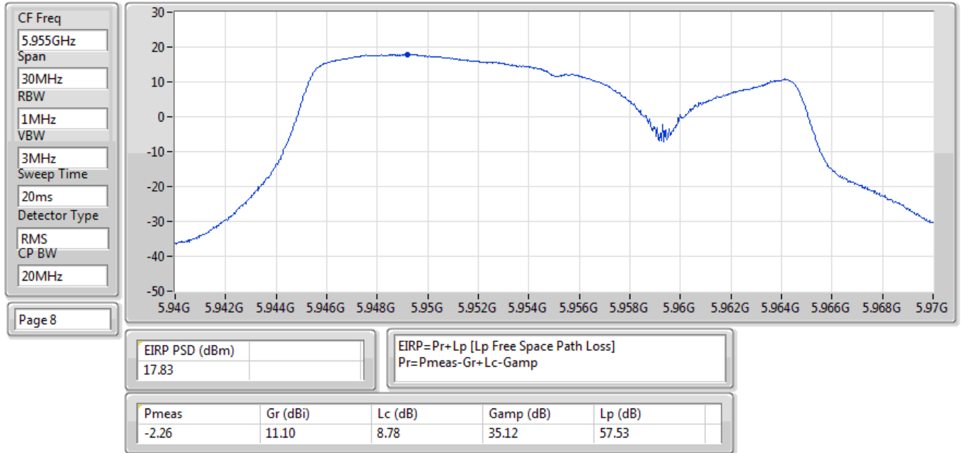
EIRP PSD;Band:6.2G;ax20;BWch:20MHz;Nss:1,(M0);Nant:4;Ch:5955MHz;TX
