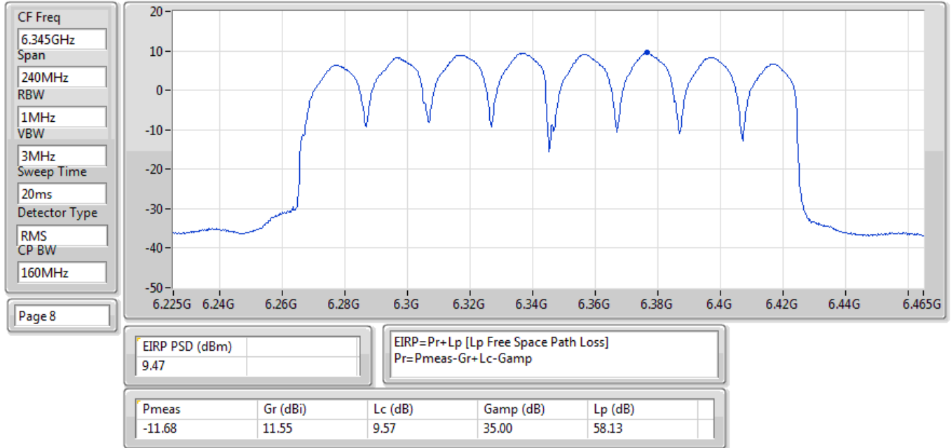
EIRP PSD;Band:6.2G;ax160;BWch:160MHz;Nss:1,(M0);Nant:4;Ch:6345MHz;TX
