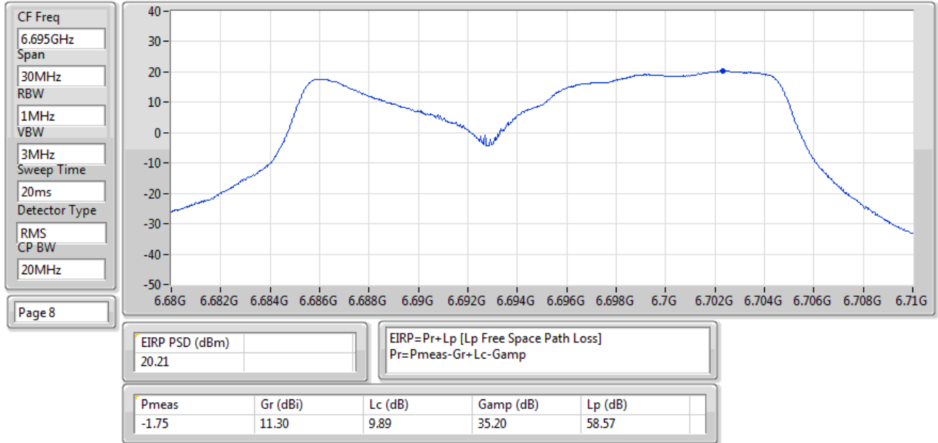
EIRP PSD;Band:6.7G;ax20;BWch:20MHz;Nss:1,(M0);Nant:4;Ch:6695MHz;TX
