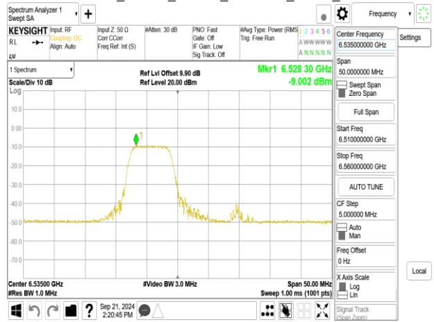
802.11be_20MHz_ChainB_6535MHz_RU106_53
