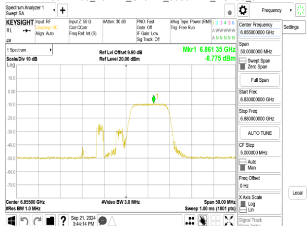
802.11be_20MHz_ChainB_6855MHz_RU106_54
