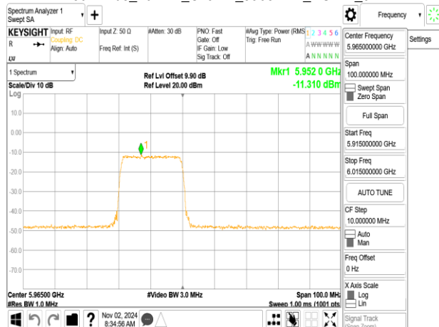
802.11be_40MHz_ChainA_5965MHz_RU242_61
