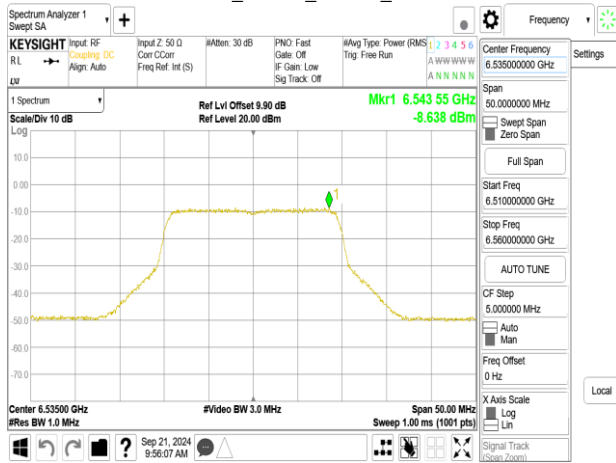
802.11be_20MHz_ChainB_6535MHz_106+26_MRUI
