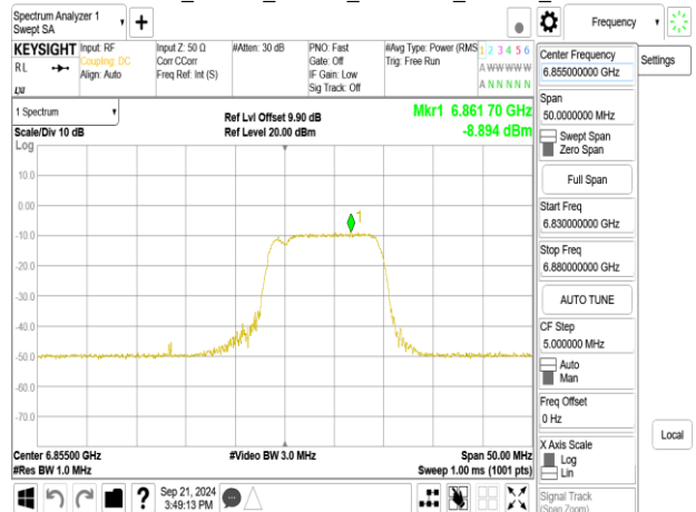
802.11be_20MHz_ChainB_6855MHz_52+26_MRU3
