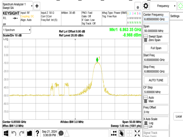
802.11be_20MHz_ChainB_6855MHz_RU52_40
