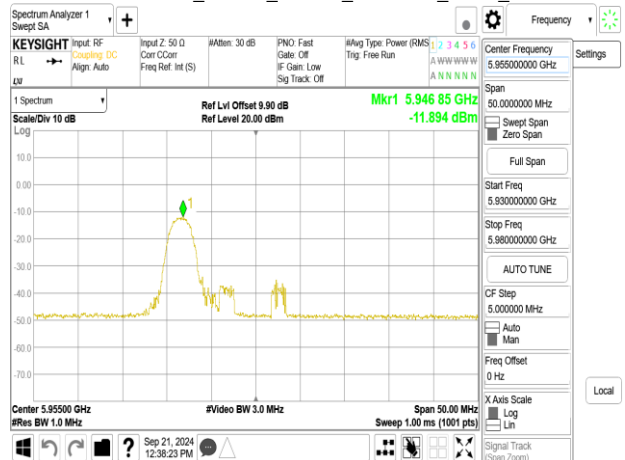
802.11be_20MHz_ChainB_5955MHz_RU52_37
