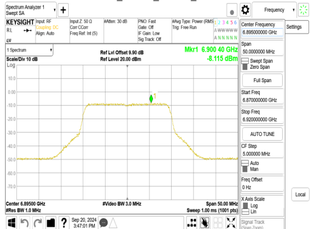
802.11be_20MHz_ChainB_6895MHz_106+26_MRU1
