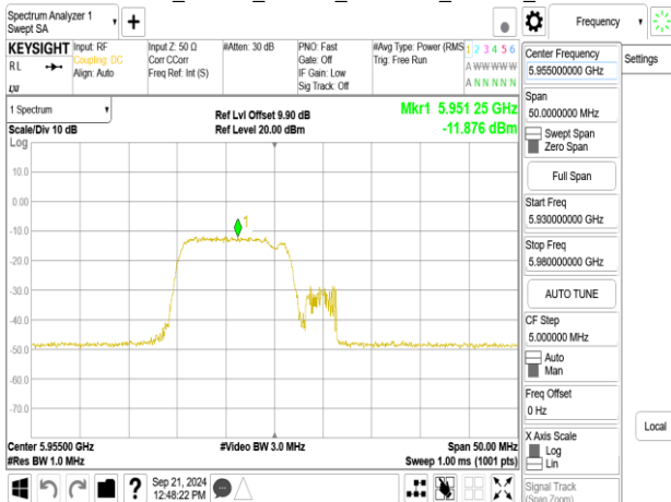
802.11be_20MHz_ChainB_5955MHz_52+26_MRUI1
