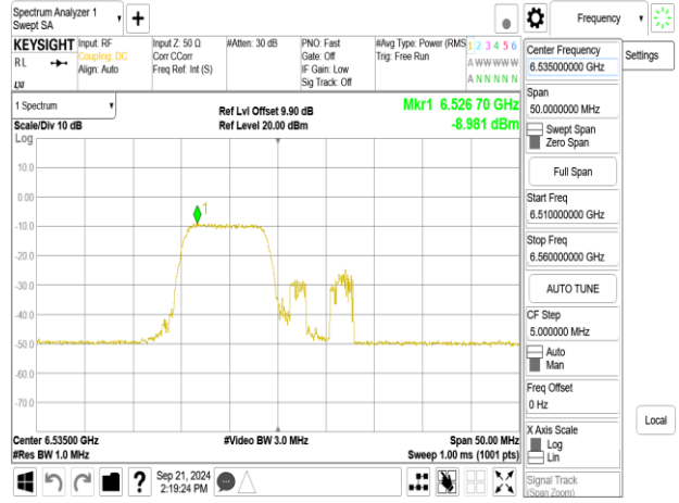
802.11be_20MHz_ChainB_6535MHz_RU26_0
