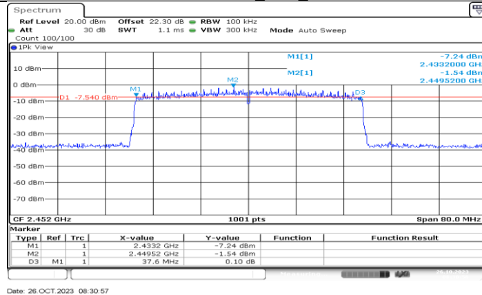
11AX40MIMO_Ant1_2452
