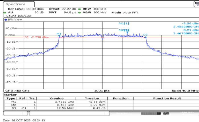
11N20MIMO_Ant1_2462
