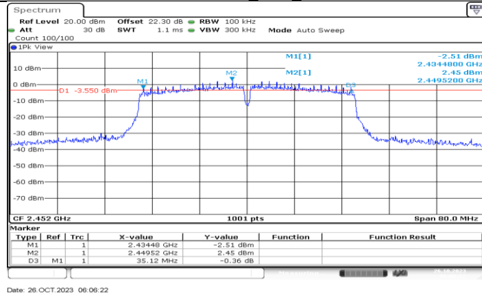
11N40MIMO_Ant1_2452
