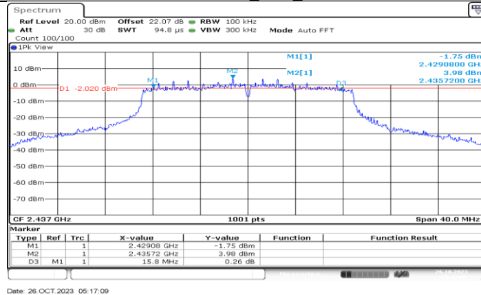
11N20MIMO_Ant0_2437
