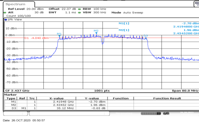
11N40MIMO_Ant0_2437
