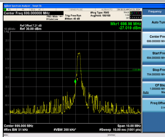
Band12-1.4MHz-QPSK-23017-1-0-Low--27.02-PASS
