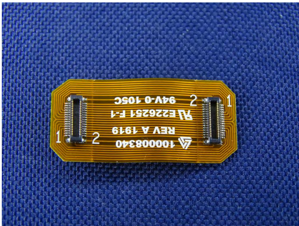
(49) EUT Photo
