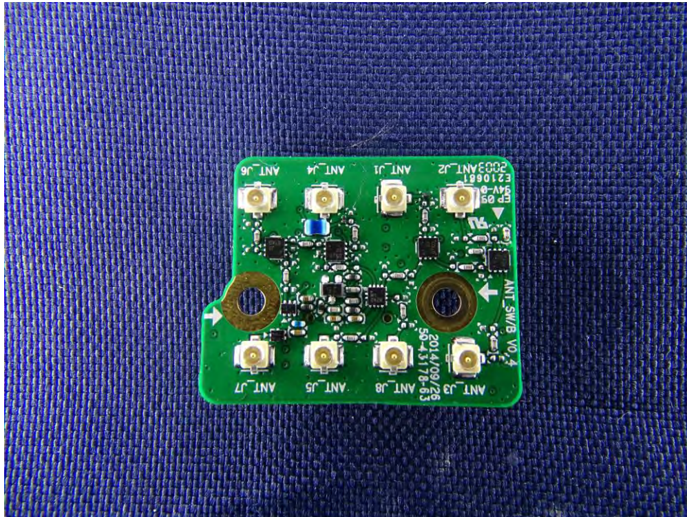
(53) EUT Photo
