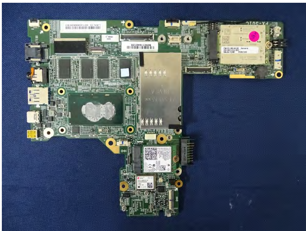
(56) EUT Photo
