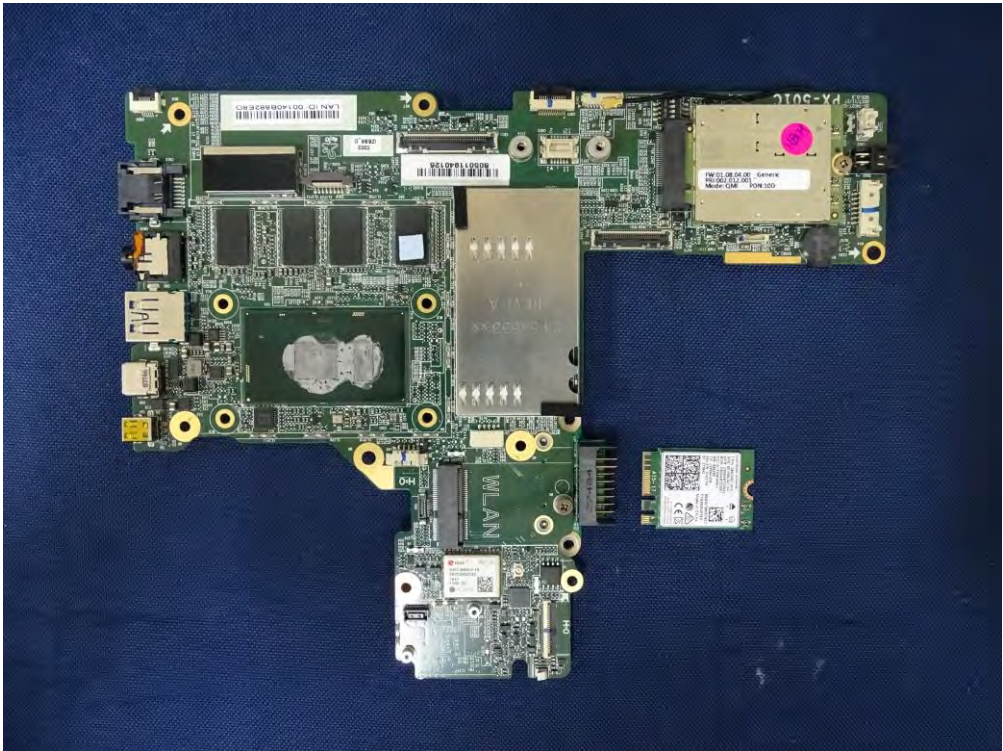
(57) EUT Photo
