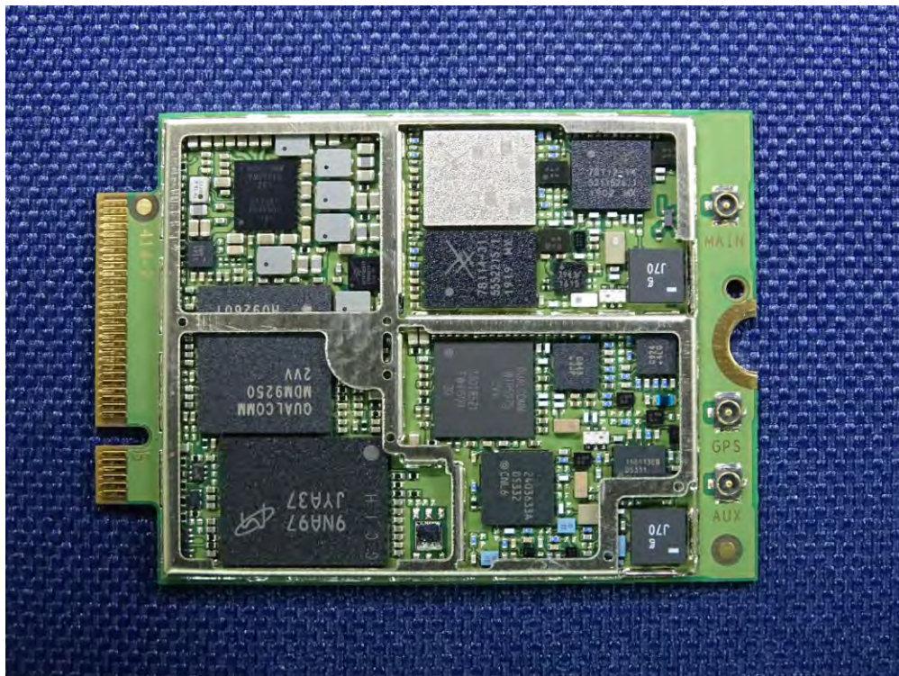
(64) EUT Photo – WWAN Module
