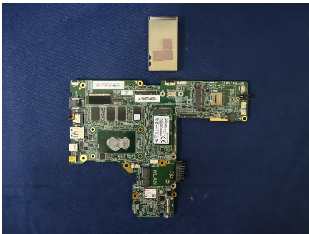
(66) EUT Photo
