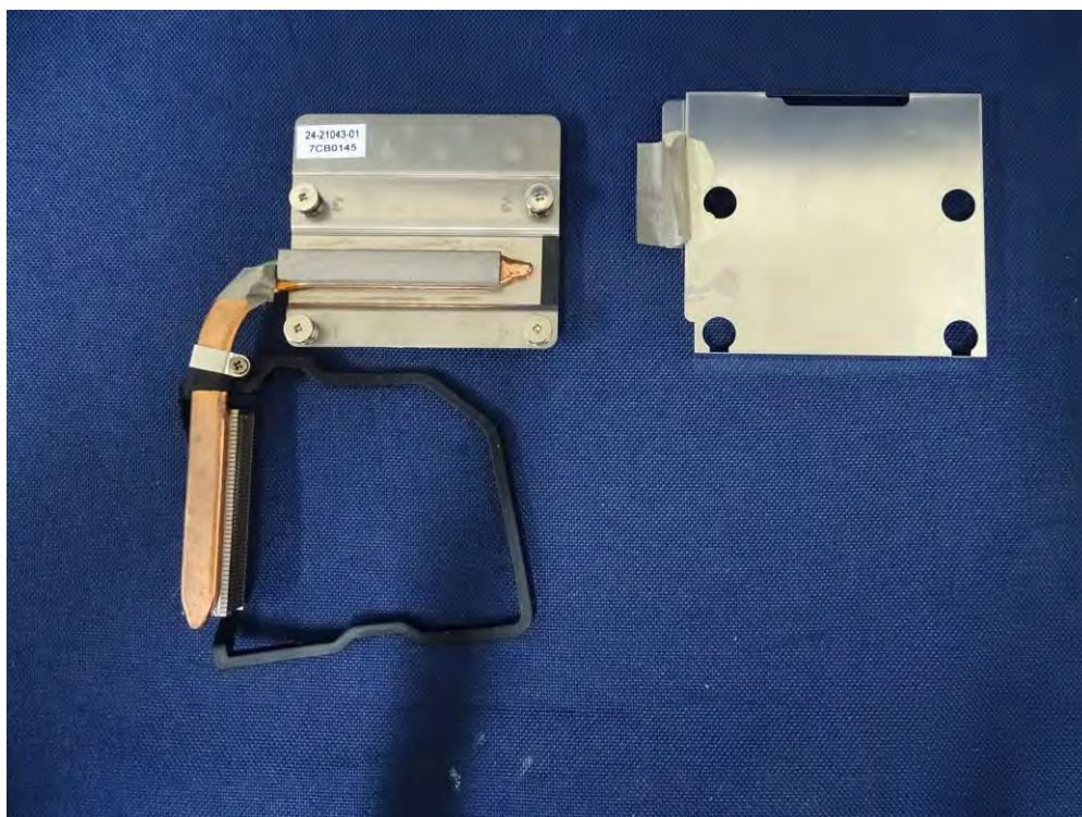
(40) EUT Photo
