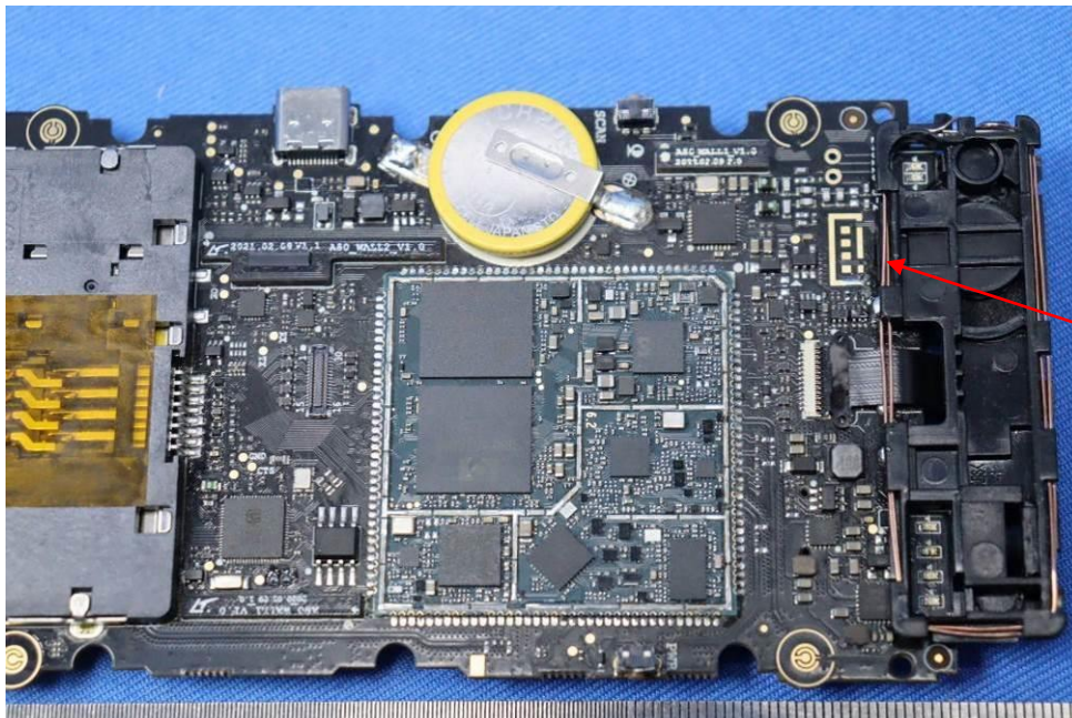
NFC Antenna
