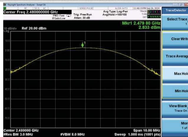
GFSK(CH78)
