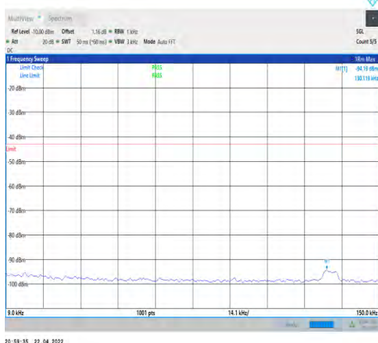
1-N66-PC3-15-40-M-1-DFT-PI2BPSK-Inner_1RB_L eft-1@1-0.009-0.15-Ant1--94.19--43-PASS
