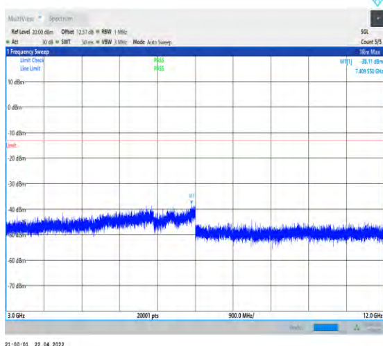
1-N66-PC3-15-40-M-1-DFT-PI2BPSK-Inner_1RB_L eft-1@1-3000-12000-Ant1--38.11--13-PASS
