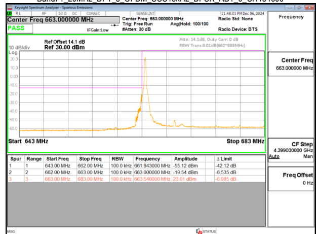
Band71 20MHz_DFT_s OFDM_SCS15kHz BPSK RB1_0_CH134600
