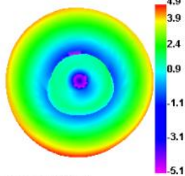
2450.000MHz
