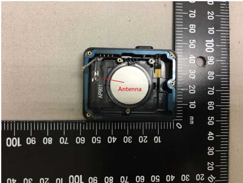
UWB Antenna
