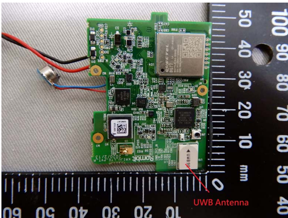
UWB Antenna
