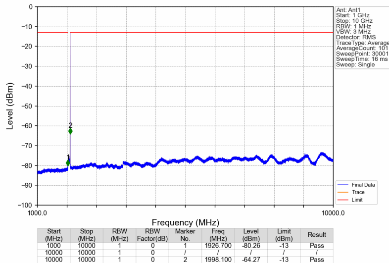
Band25_1994.9MHz_GMSK_SISO_Ant1_NTNV
