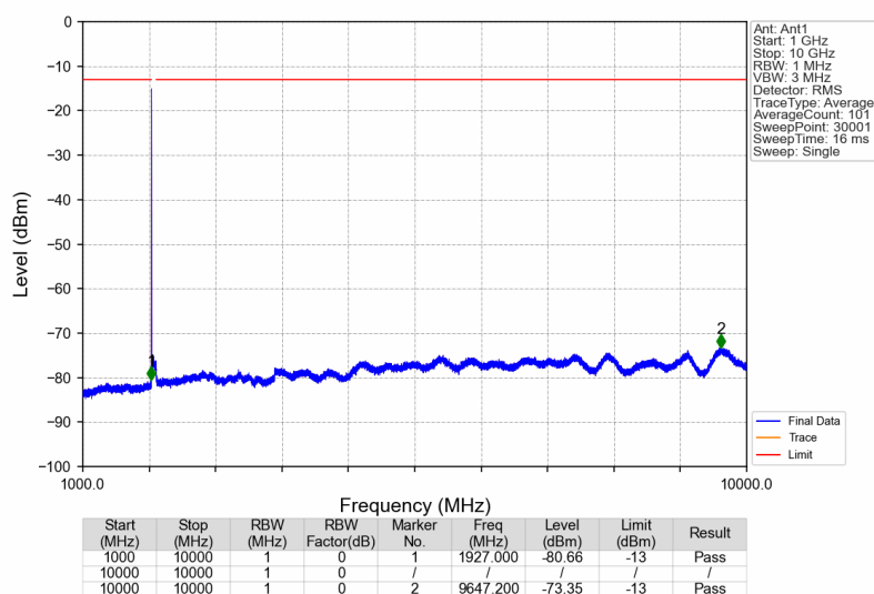
Band25_1930.1MHz_GMSK_SISO_Ant1_NTNV
