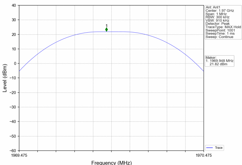
Band25_1969.975MHz_GMSK_SISO_Ant1_NTNV_AGC+3
