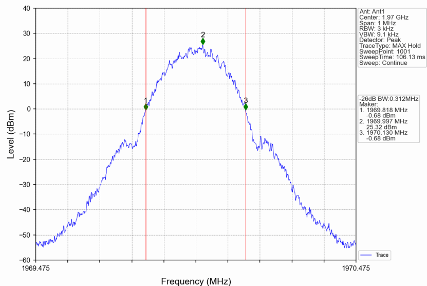
Band25_1969.975MHz_GMSK_SISO_Ant1_NTNV_AGC
