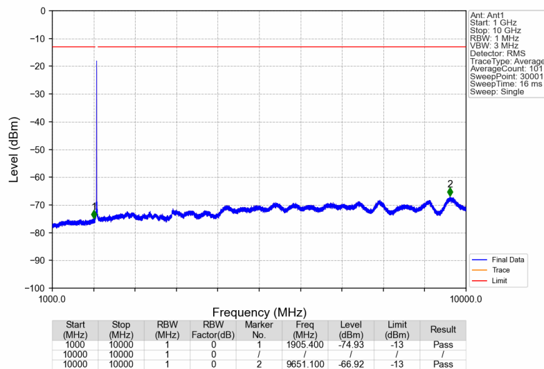
Band25_1962.5MHz_AWGN_SISO_Ant1_NTNV
