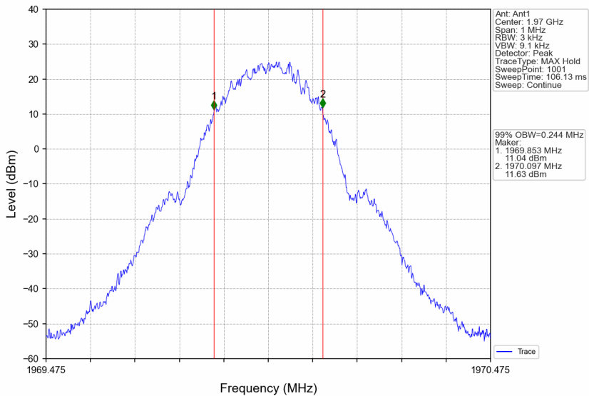
Band25_1969.975MHz_GMSK_SISO_Ant1_NTNV_AGC
