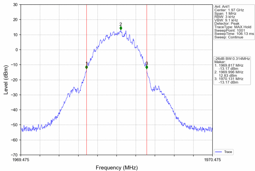
Band25_1969.975MHz_GMSK_SISO_Ant1_NTNV_AGC+3
