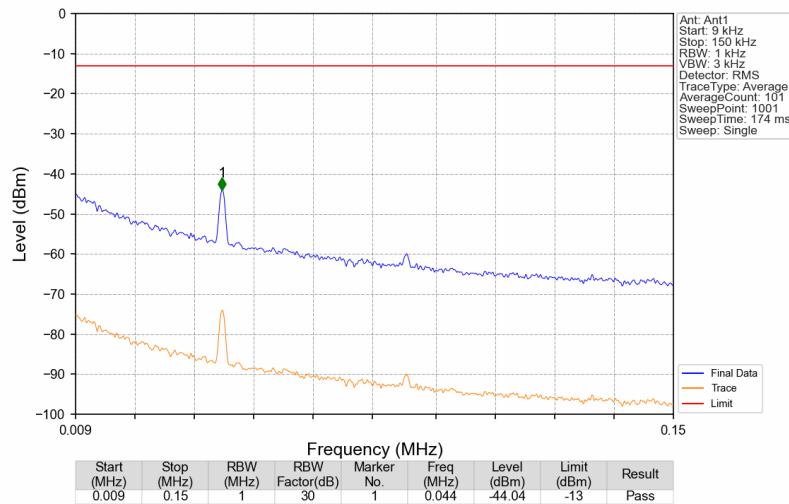
Band25_1962.5MHz_GMSK_SISO_Ant1_NTNV
