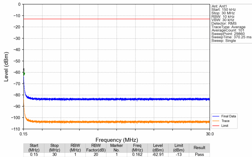
Band25_1930.1MHz_GMSK_SISO_Ant1_NTNV
