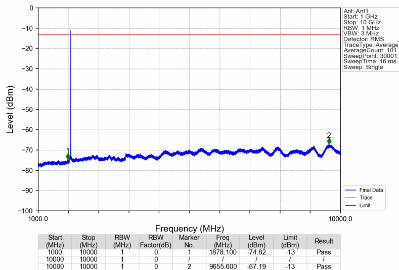
Band25_1962.5MHz_GMSK_SISO_Ant1_NTNV
