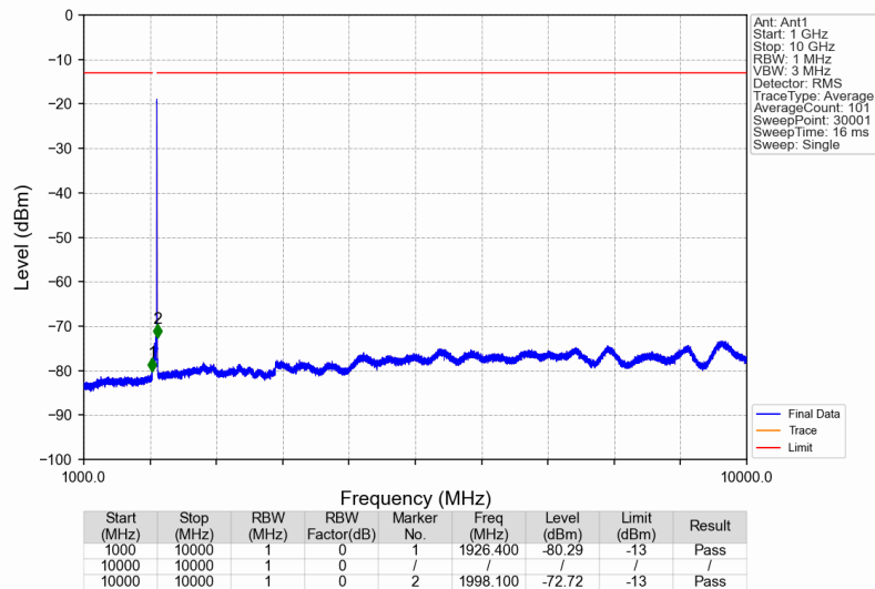
Band25_1992.5MHz_AWGN_SISO_Ant1_NTNV
