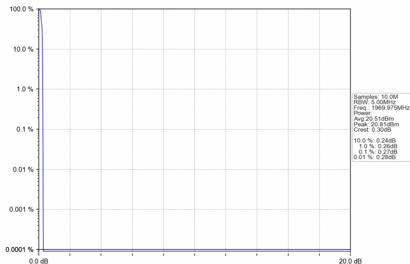
Band25_1969.975MHz_GMSK_SISO_Ant1_NTNV_AGC
