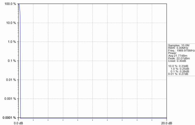
Band25_1969.975MHz_GMSK_SISO_Ant1_NTNV_AGC+3
