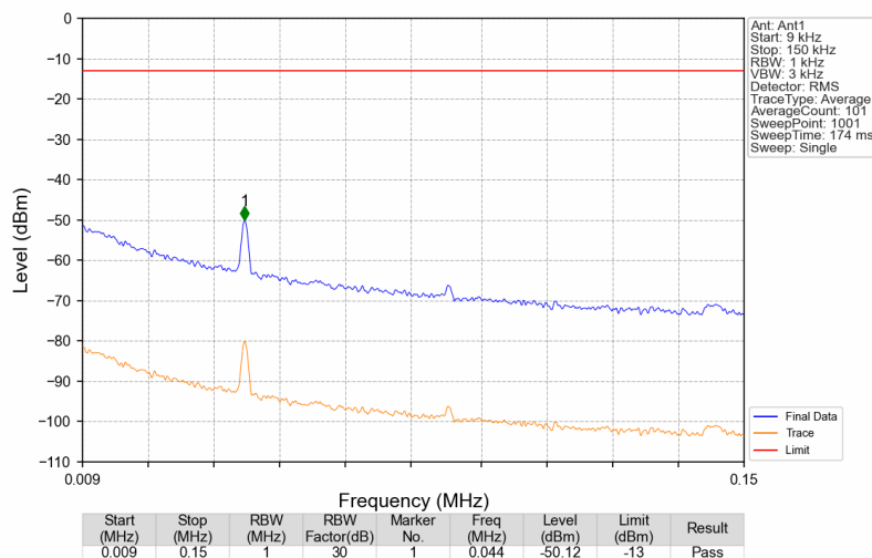
Band25_1932.5MHz_AWGN_SISO_Ant1_NTNV
