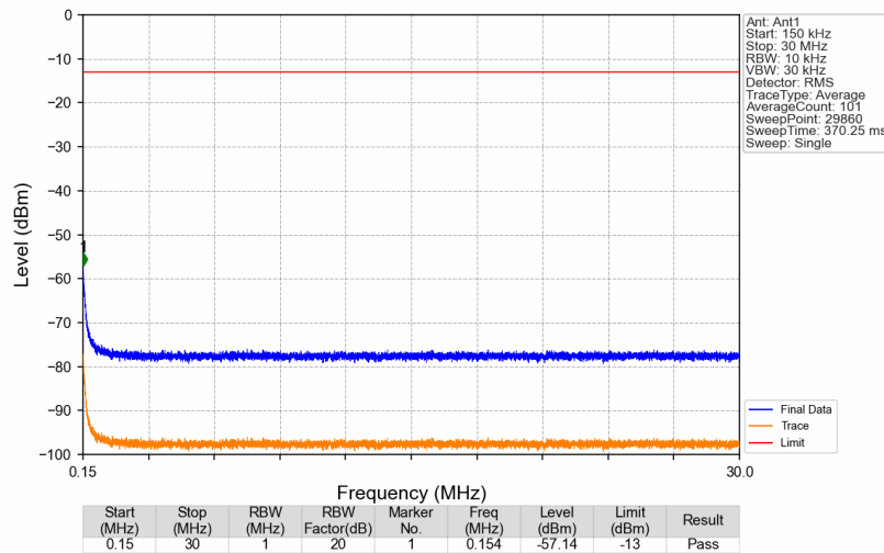
Band25_1962.5MHz_GMSK_SISO_Ant1_NTNV
