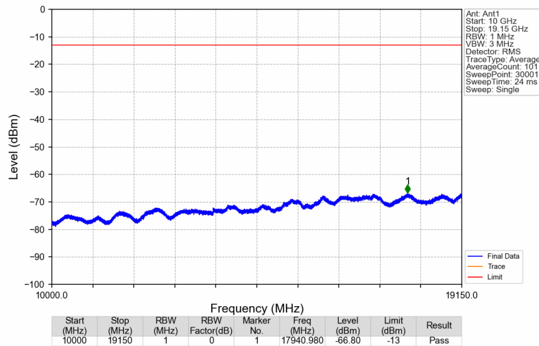
Band25_1992.5MHz_AWGN_SISO_Ant1_NTNV
