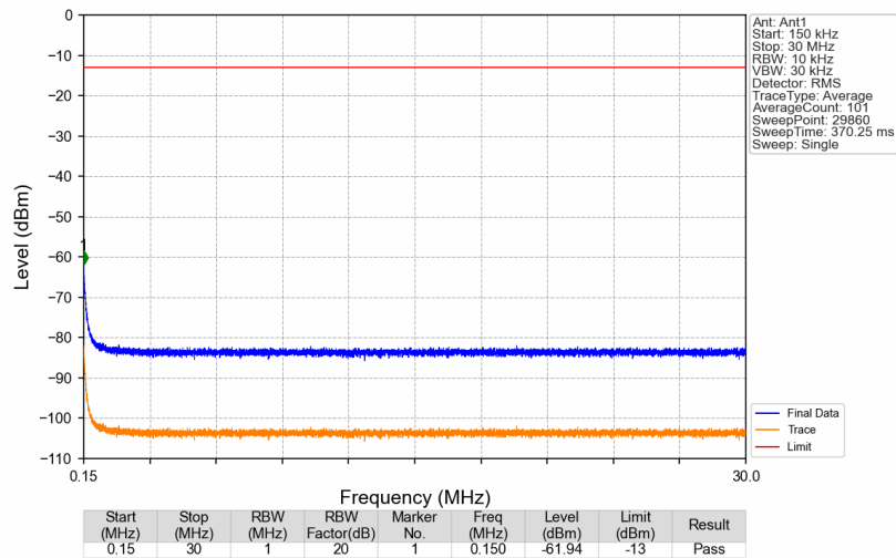
Band25_1994.9MHz_GMSK_SISO_Ant1_NTNV
