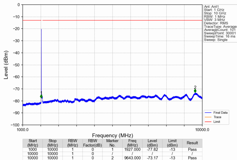
Band25_1932.5MHz_AWGN_SISO_Ant1_NTNV
