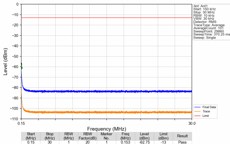
Band25_1932.5MHz_AWGN_SISO_Ant1_NTNV
