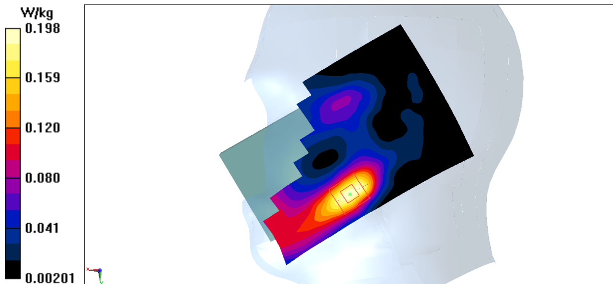
Fig.9 LTE Band7
