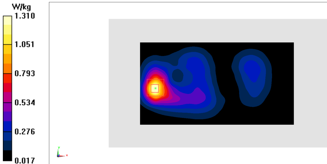
Fig.8 WCDMA1900
