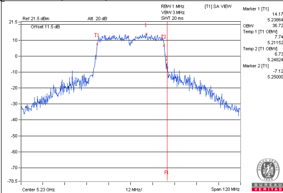
802.11ac(VHT40)_Chain3 / CH46
