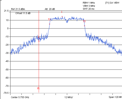
802.11ac(VHT40)_Chain3 / CH151
