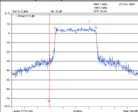
802.11ac(VHT80)_Chain3 / CH155
