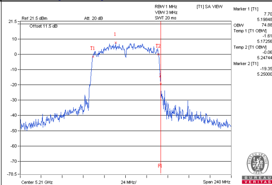
802.11ac(VHT80)_Chain3 / CH42
