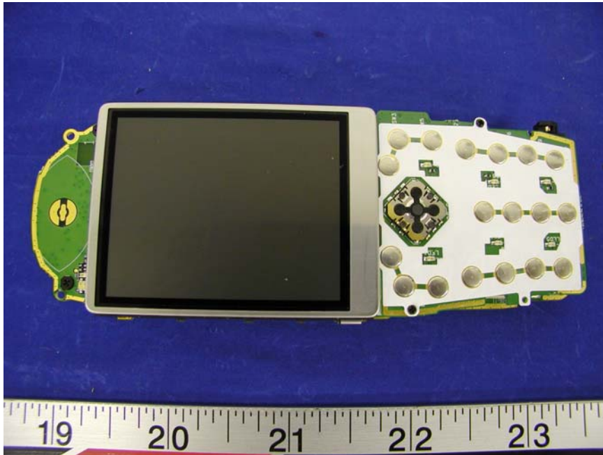
EUT SV10A/SV10B – LCD Display View
