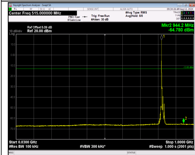
5-5-5MHz-3MHz-QPSK-QPSK-20425-20464-1RB#0-0RB #0-30~1000MHz-PASS
