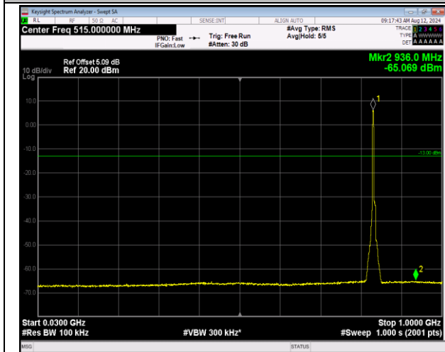
5-5-3MHz-5MHz-QPSK-QPSK-20501-20540-15RB#0-25 RB#0-30~1000MHz-PASS
