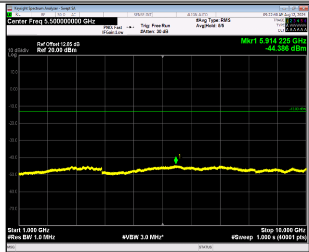
5-5-3MHz-5MHz-QPSK-QPSK-20586-20625-15RB#0-25RB #0-1000~10000MHz-PASS
