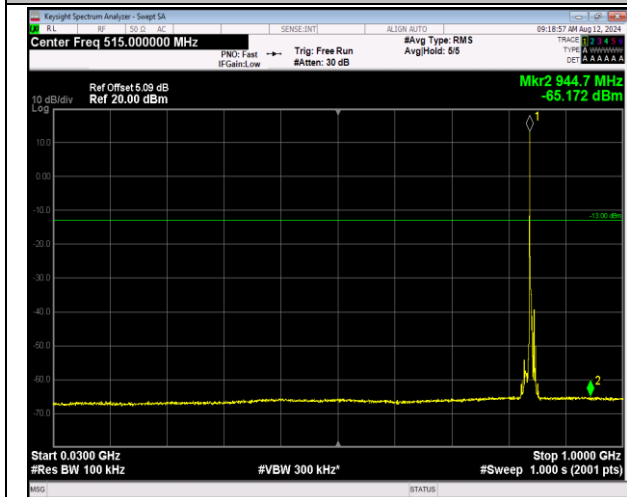
5-5-3MHz-5MHz-QPSK-QPSK-20586-20625-1RB#0-ORB #0-30~1000MHz-PASS
