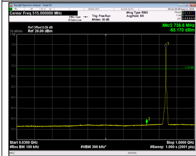
5-5-3MHz-5MHz-QPSK-QPSK-20586-20625-15RB#0-25 RB#0-30~1000MHz-PASS
