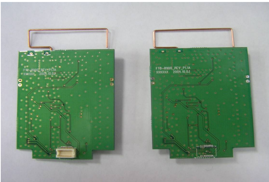
900MHz RX Bottom side
