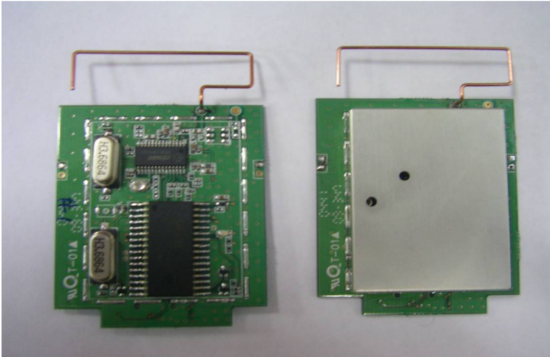
900MHz RX Top side
