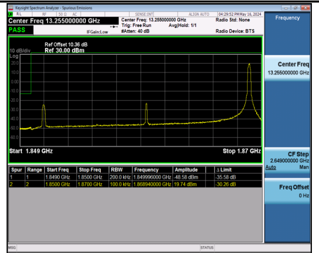
Band2_20MHz_QPSK_18700_1RB#99
