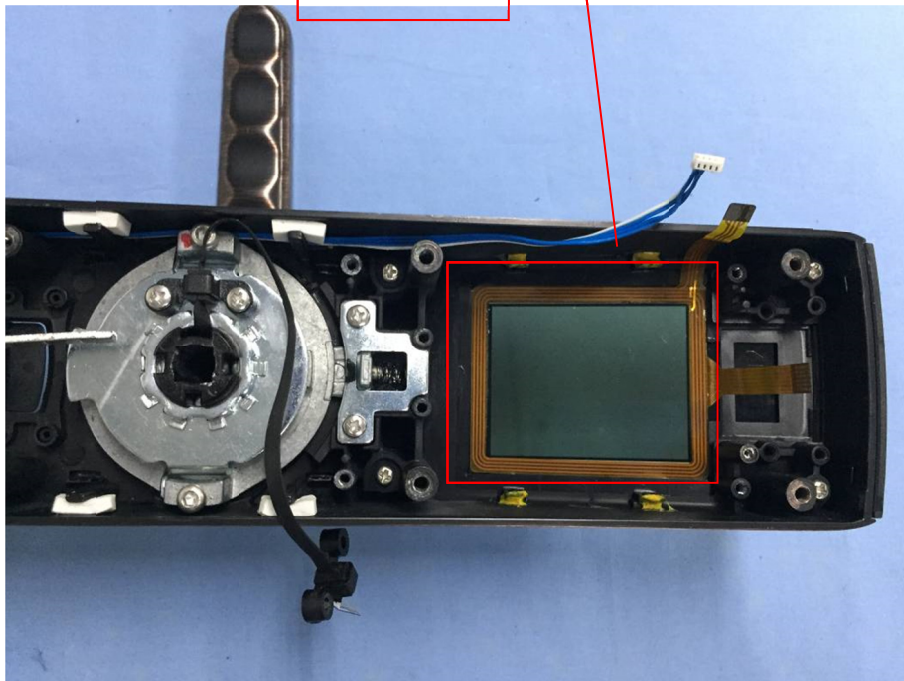
NFC Antenna
