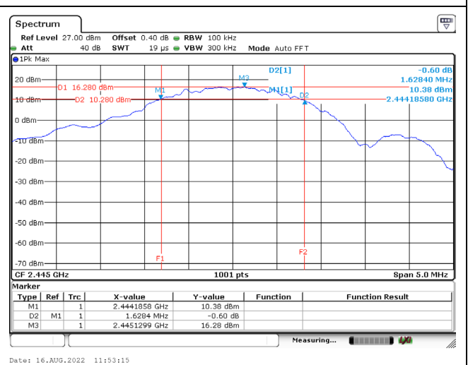
O-QPSK / 2445 MHz
