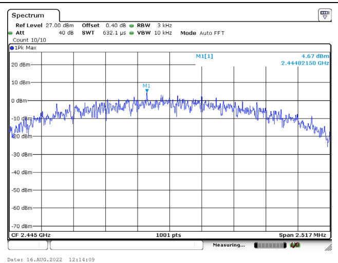
O-QPSK / 2445 MHz
