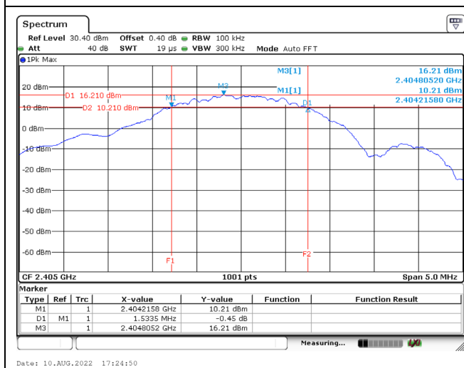
O-QPSK / 2405 MHz
