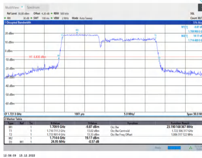
66-66-10MHz-15MHz-QPSK-QPSK-132351-132471-50RB#0-75RB#0
