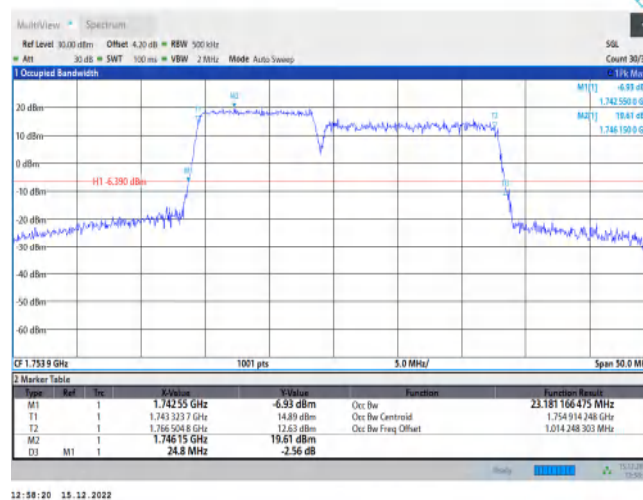
66-66-10MHz-15MHz-QPSK-QPSK-132351-132471-50RB#0-75RB#0
