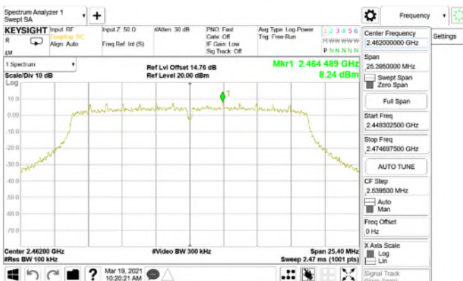
Reference Level_802.11n_20MHz_Chain0_2462MHz
