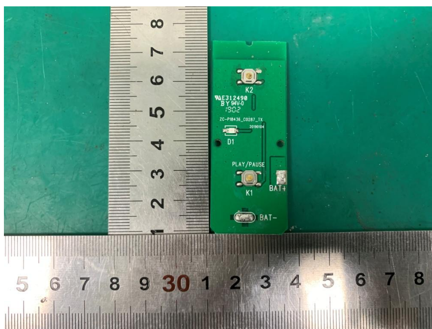
EUT-10
