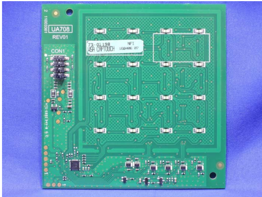
(18) EUT Photo
