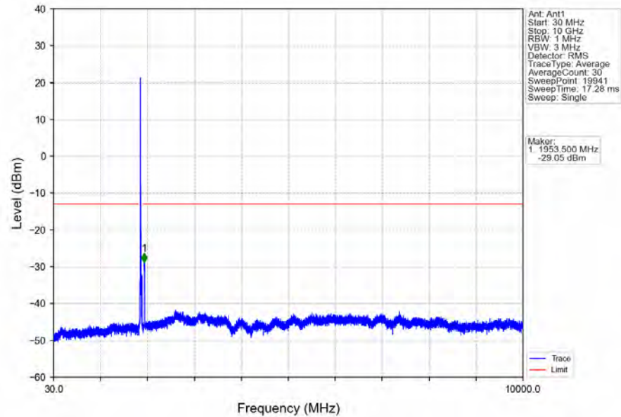
Band2_20MHz_16QAM_MCH_1880MHz_RB_1_0_NTNV
