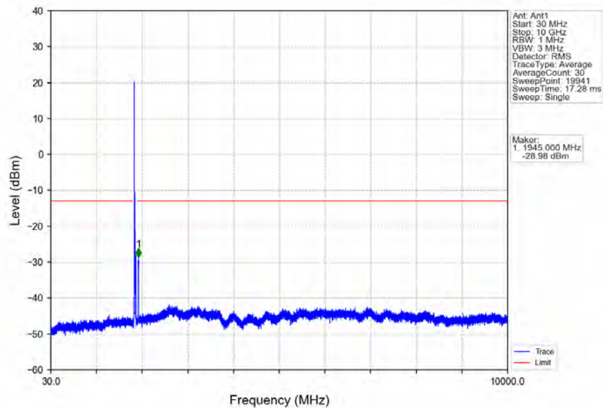
Band2_20MHz_64QAM_LCH_1860MHz_RB_1_0_NTNV
