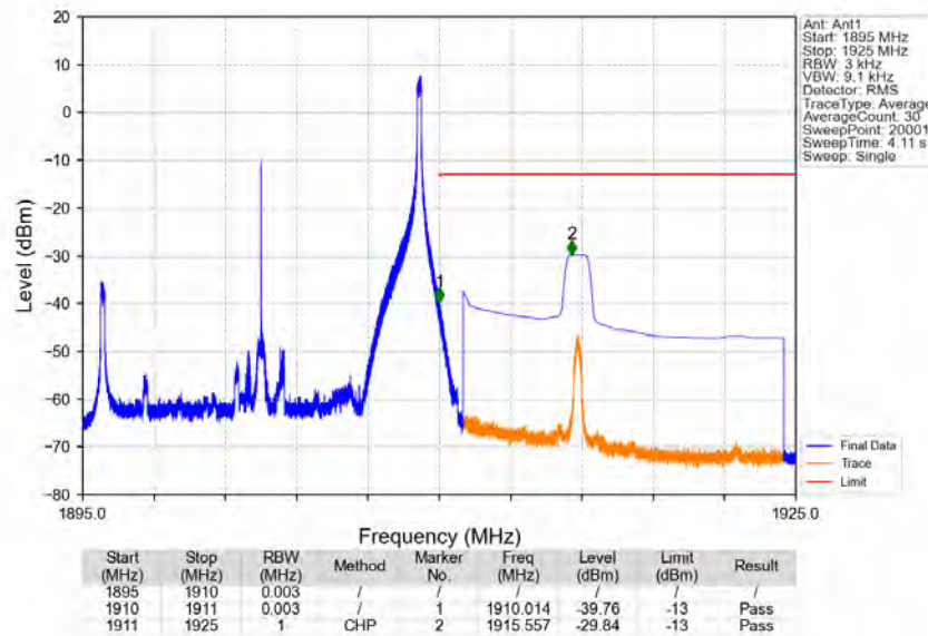
Band2_15MHz_16QAM_HCH_1902.5MHz_RB_1_74_NTNV
