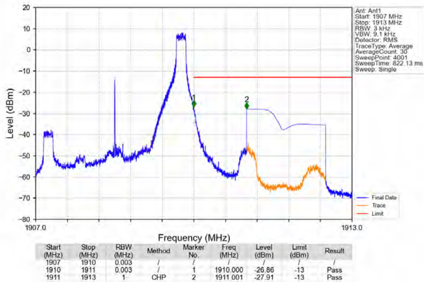
Band2_3MHz_QPSK_HCH_1908.5MHz_RB_1_14_NTNV
