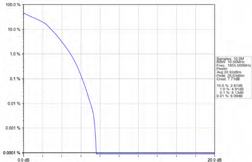
Band2_10MHz_16QAM_LCH_1855MHz_RB_50_0_NTNV
