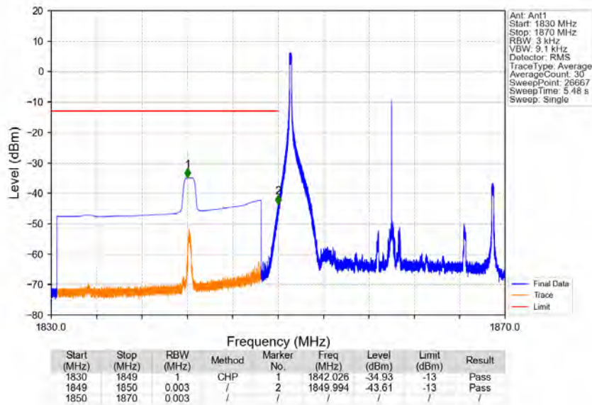
Band2_20MHz_16QAM_LCH_1860MHz_RB_1_0_NTNV
