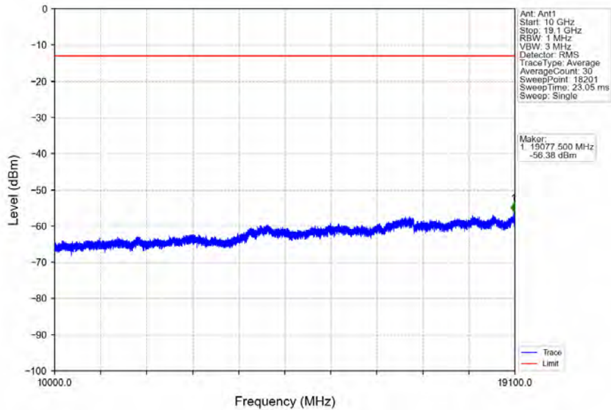
Band2_10MHz_16QAM_LCH_1855MHz_RB_50_0_NTNV
