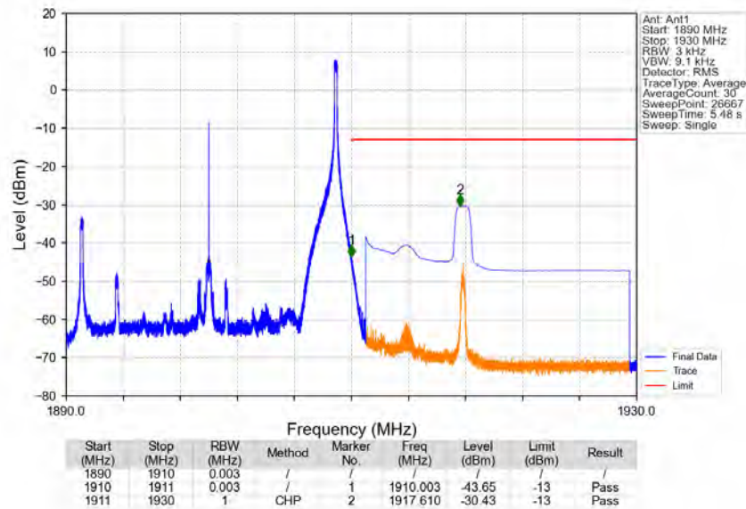
Band2_20MHz_QPSK_HCH_1900MHz_RB_1_99_NTNV
