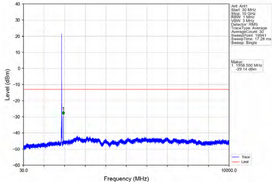
Band2_10MHz_16QAM_MCH_1880MHz_RB_1_0_NTNV
