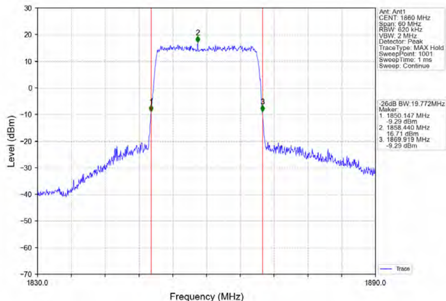
Band2_20MHz_64QAM_LCH_1860MHz_RB_100_0_NTNV
