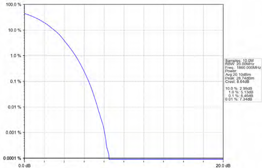
Band2_20MHz_64QAM_LCH_1860MHz_RB_100_0_NTNV
