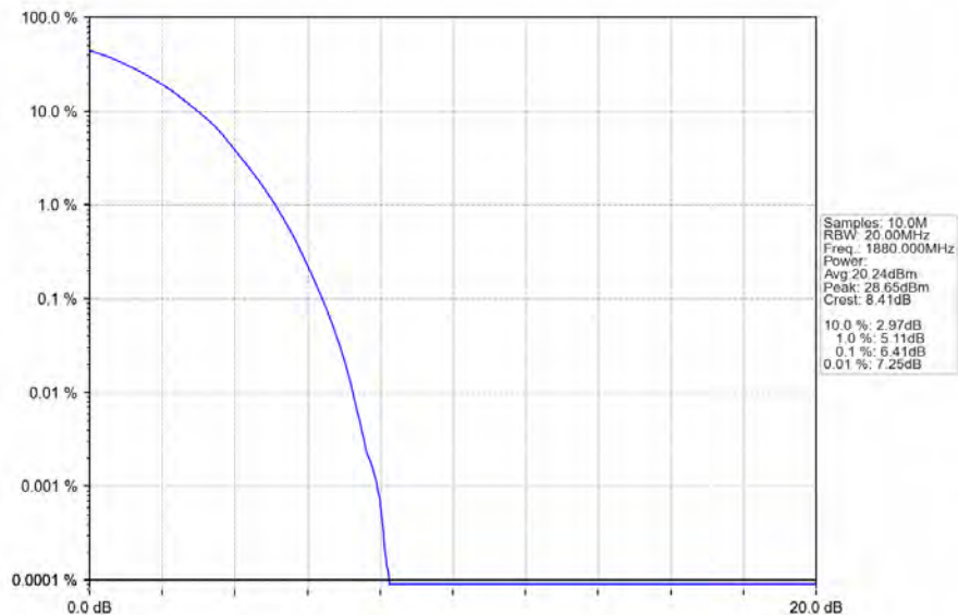
Band2_20MHz_64QAM_MCH_1880MHz_RB_100_0_NTNV
