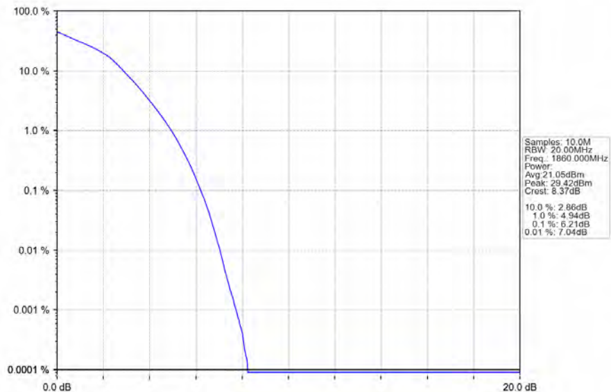
Band2_20MHz_16QAM_LCH_1860MHz_RB_100_0_NTNV
