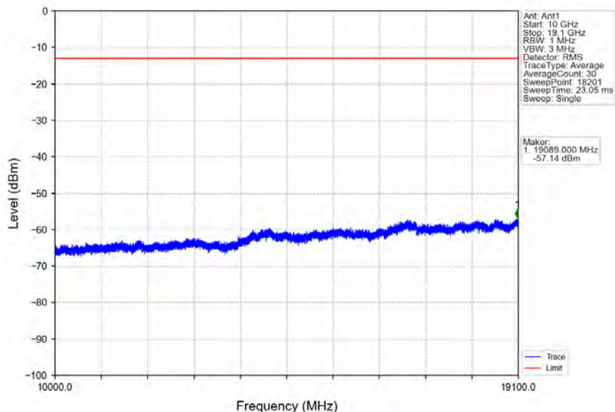
Band2_20MHz_QPSK_HCH_1900MHz_RB_1_0_NTNV
