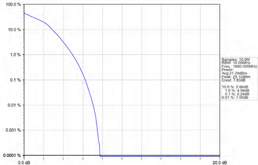
Band2_10MHz_16QAM_MCH_1880MHz_RB_50_0_NTNV
