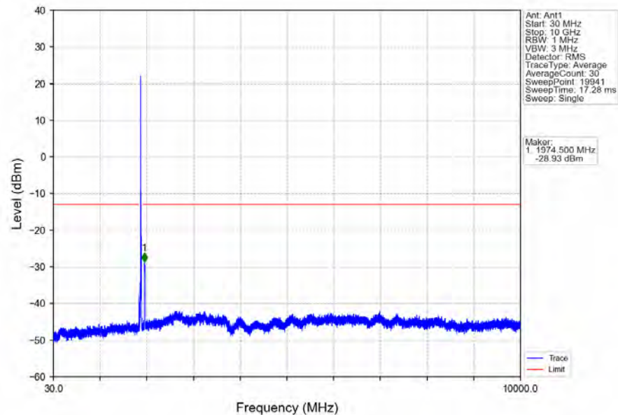
Band2_20MHz_QPSK_HCH_1900MHz_RB_1_0_NTNV
