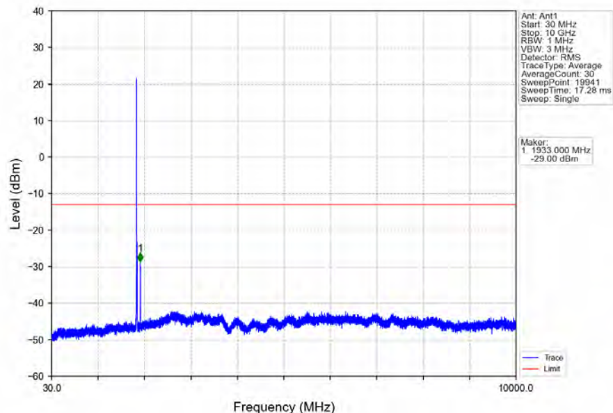
Band2_10MHz_16QAM_LCH_1855MHz_RB_1_0_NTNV
