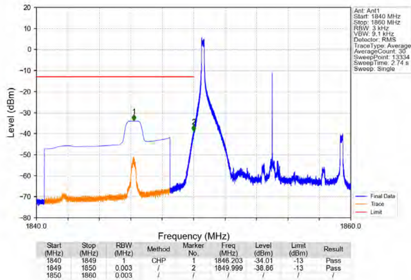
Band2_10MHz_64QAM_LCH_1855MHz_RB_1_0_NTNV
