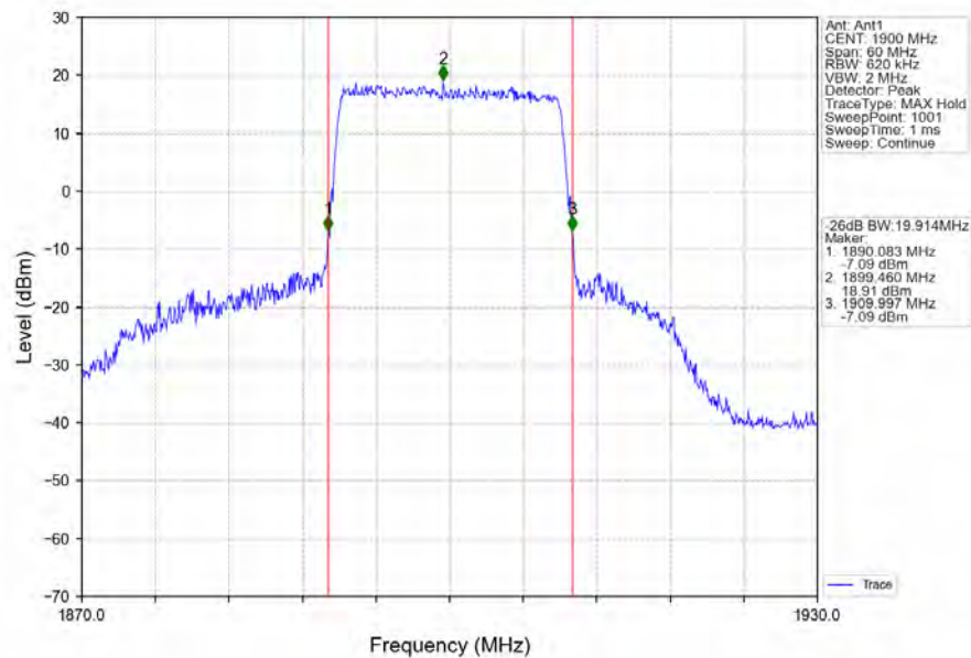
Band2_20MHz_QPSK_HCH_1900MHz_RB_100_0_NTNV
