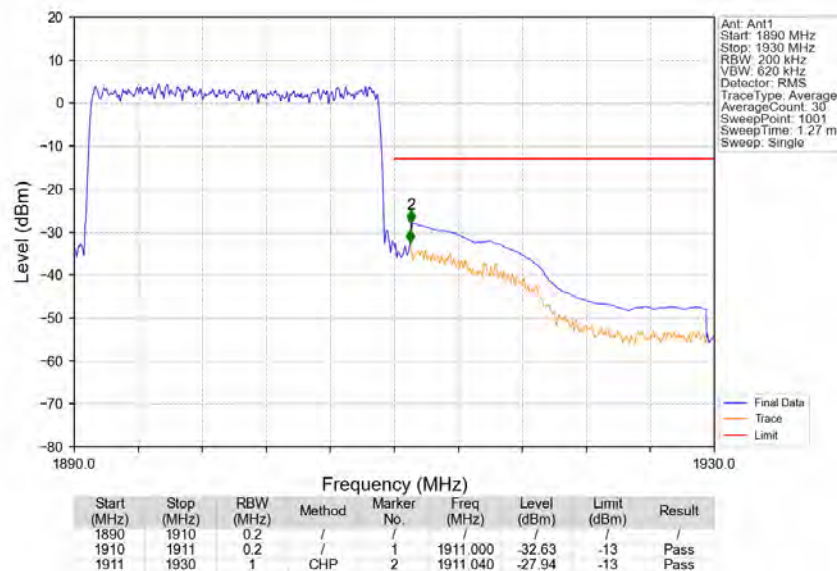
Band2_20MHz_16QAM_HCH_1900MHz_RB_100_0_NTNV
