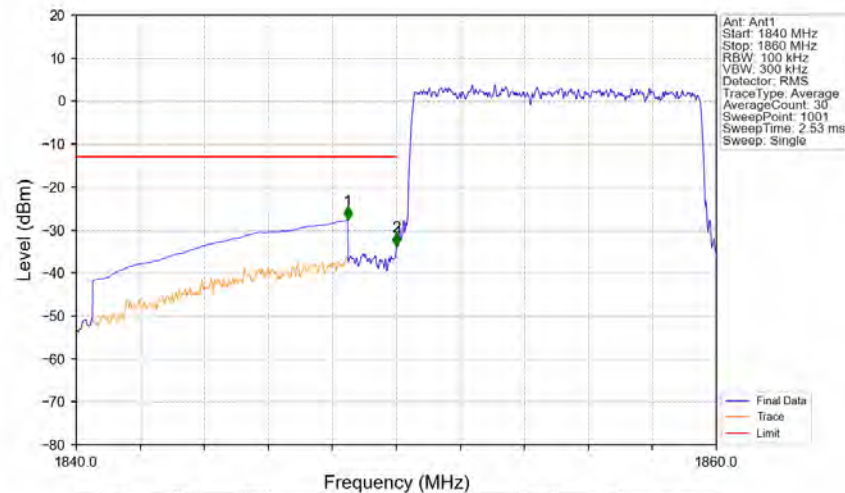
Band2_10MHz_16QAM_LCH_1855MHz_RB_50_0_NTNV
