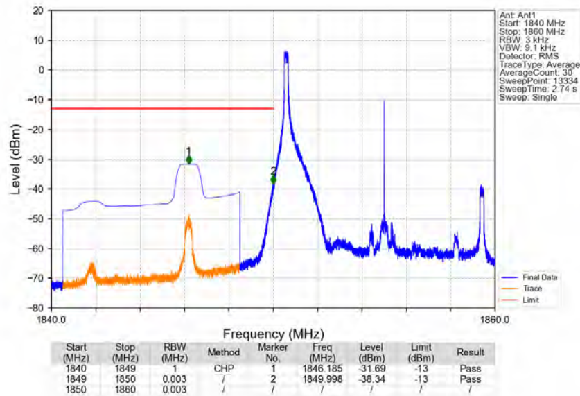
Band2_10MHz_16QAM_LCH_1855MHz_RB_1_0_NTNV
