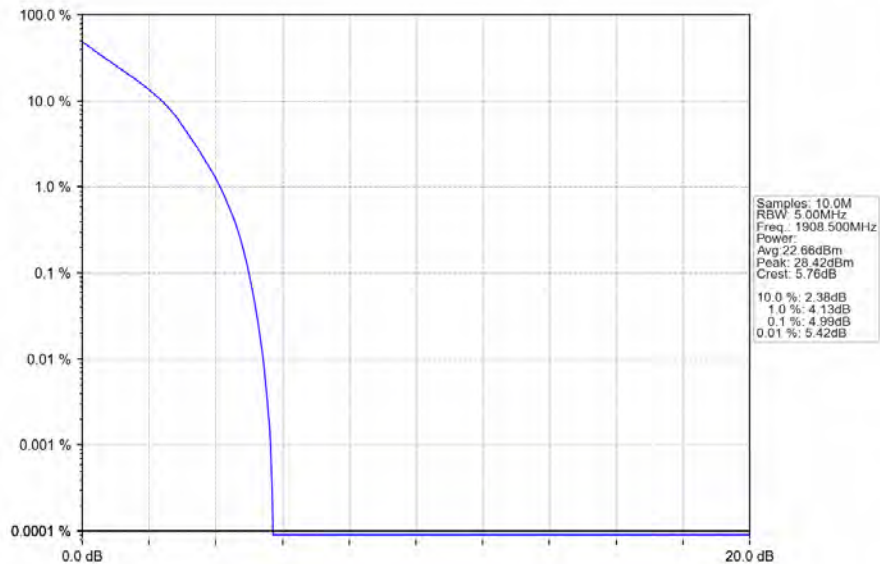
Band2_3MHz_QPSK_HCH_1908.5MHz_RB_15_0_NTNV
