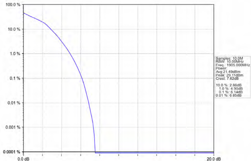
Band2_10MHz_16QAM_HCH_1905MHz_RB_50_0_NTNV
