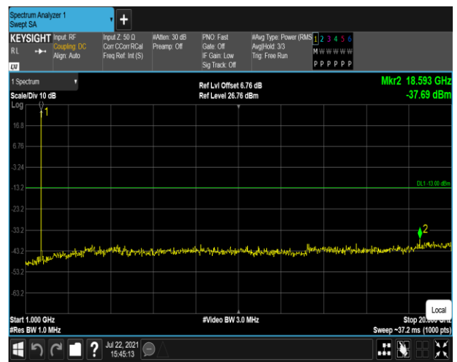
Band4-1.4MHz-QPSK-20175:1000~20000MHz
