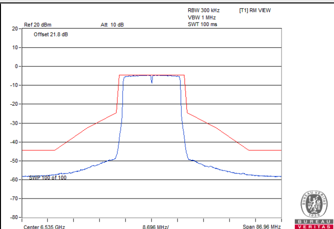
802.11ax (HE20) CDD / Chain 1 : CH 117
