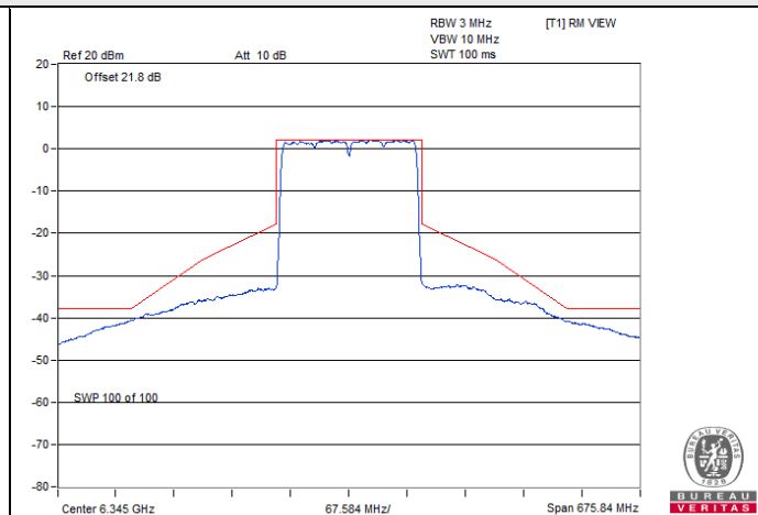
802.11ax (HE160) CDD / Chain 1 : CH 79
