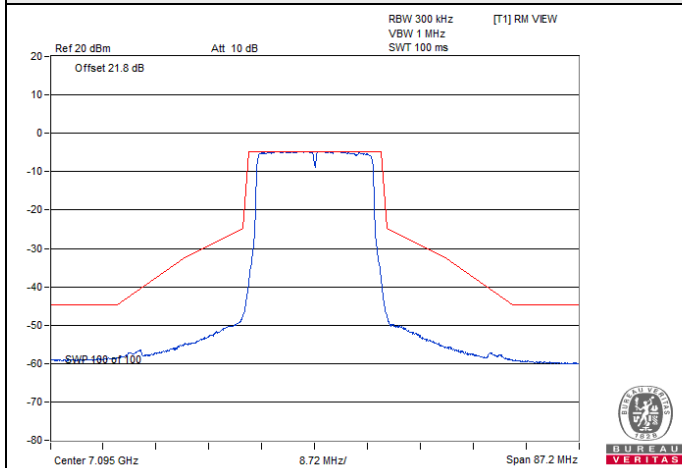
802.11ax (HE20) CDD / Chain 1 : CH 229
