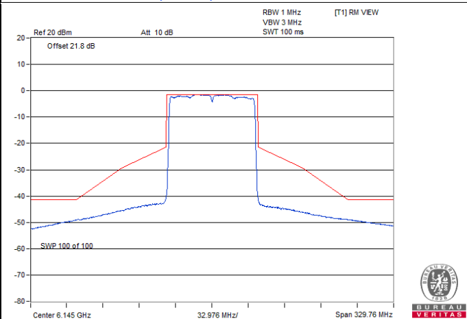
802.11ax (HE80) CDD / Chain 1 : CH 39
