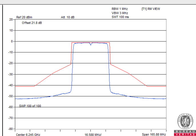
802.11ax (HE40) CDD / Chain 0 : CH 59
