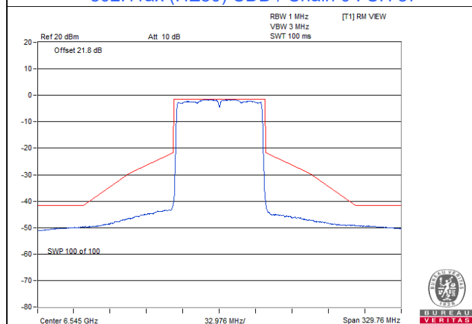
802.11ax (HE80) CDD / Chain 0 : CH 119
