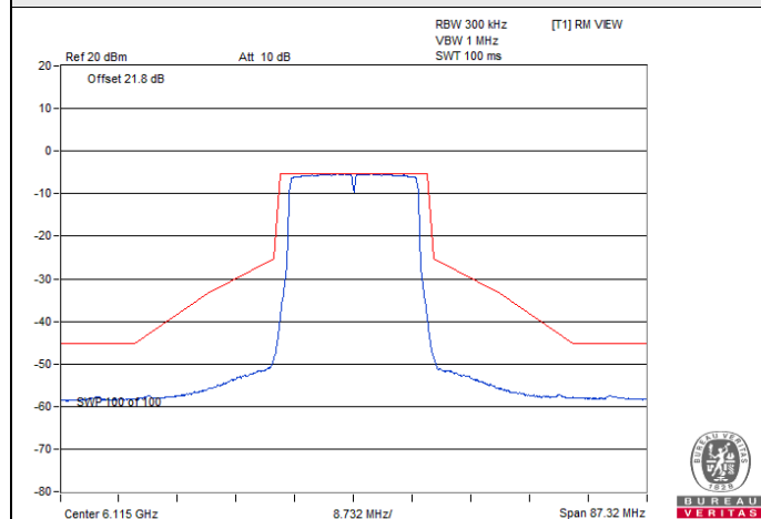
802.11ax (HE20) CDD / Chain 0 : CH 33
