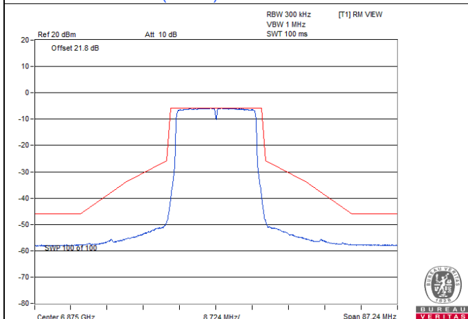
802.11ax (HE20) CDD / Chain 1 : CH 185
