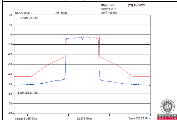
802.11ax (HE80) CDD / Chain 0 : CH 87
