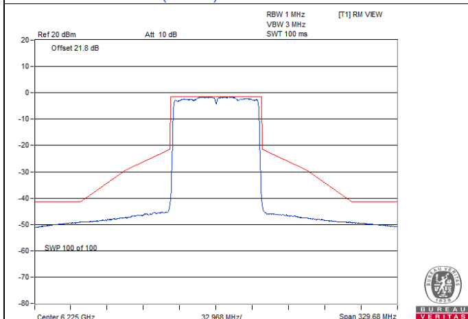
802.11ax (HE80) CDD / Chain 1 : CH 55
