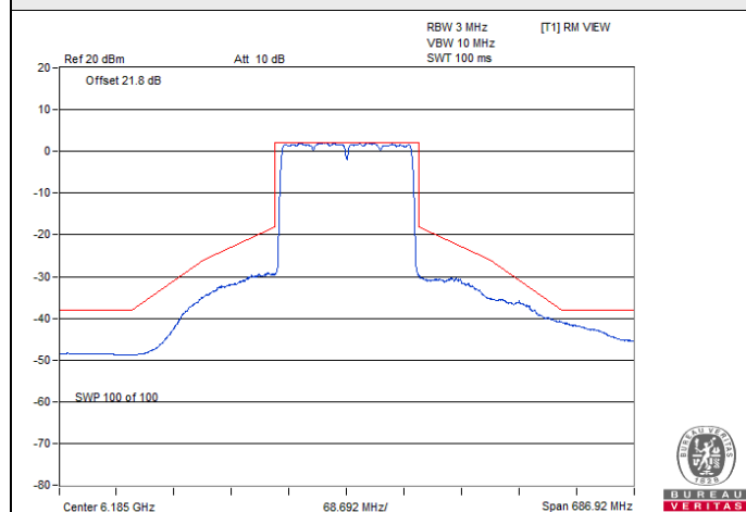
802.11ax (HE160) CDD / Chain 0 : CH 47
