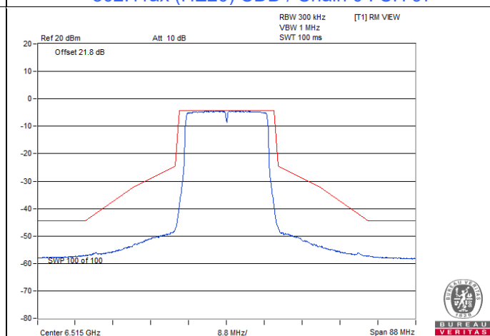
802.11ax (HE20) CDD / Chain 0 : CH 113
