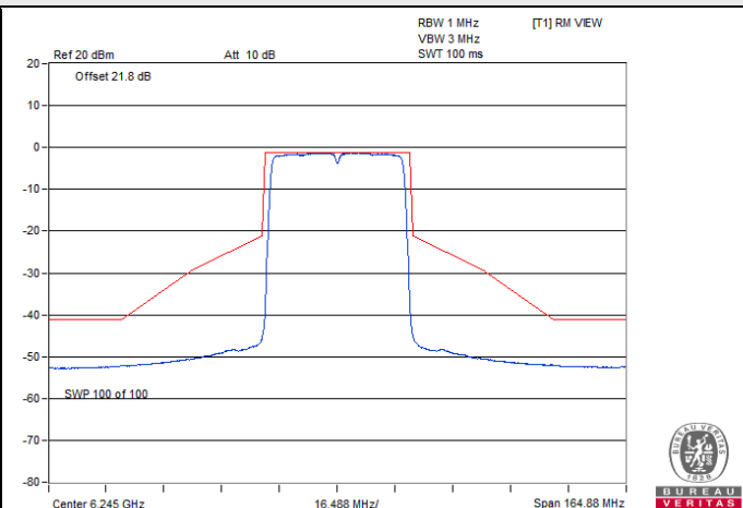
802.11ax (HE40) CDD / Chain 1 : CH 59
