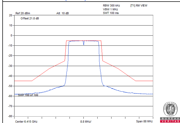
802.11ax (HE20) CDD / Chain 0 : CH 93
