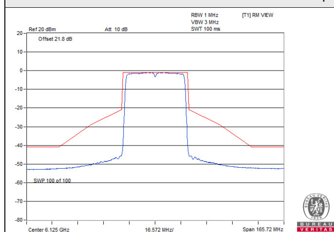
802.11ax (HE40) CDD / Chain 0 : CH 35
