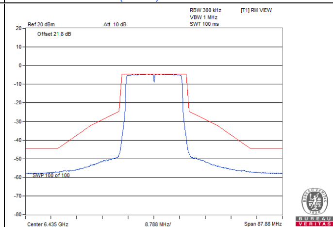
802.11ax (HE20) CDD / Chain 0 : CH 97
