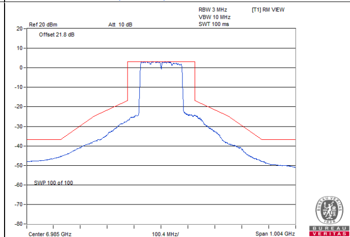
802.11ax (HE160) CDD / Chain 1 : CH 207
