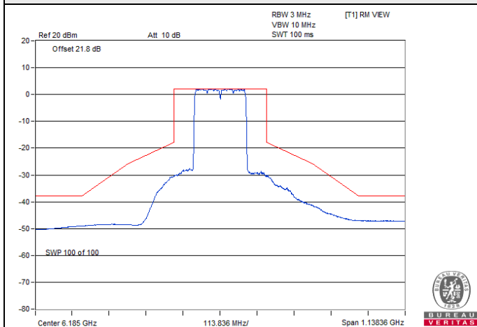
802.11ax (HE160) CDD / Chain 1 : CH 47
