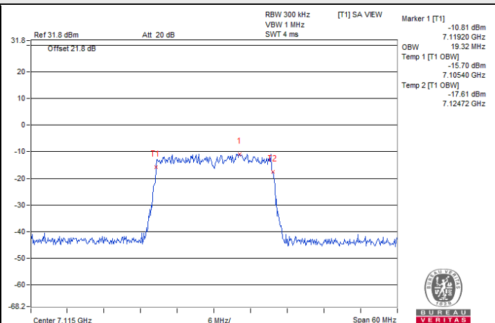
802.11ax (HE20) / Chain 1 : CH 233
