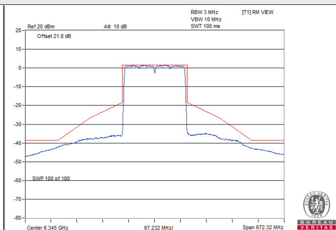
802.11ax (HE160) CDD / Chain 0 : CH 79
