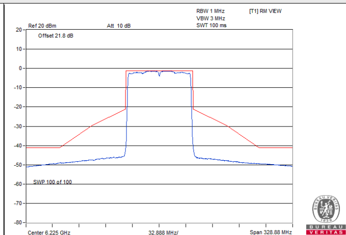
802.11ax (HE80) CDD / Chain 0 : CH 55
