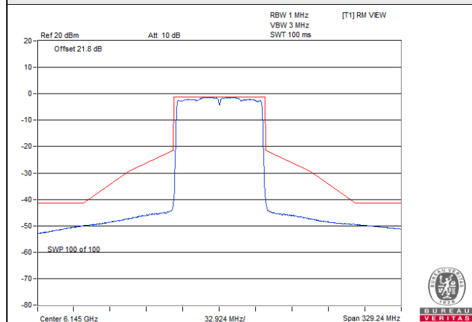
802.11ax (HE80) CDD / Chain 0 : CH 39
