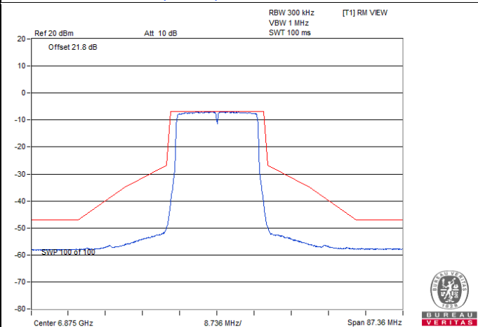
802.11ax (HE20) CDD / Chain 0 : CH 185
