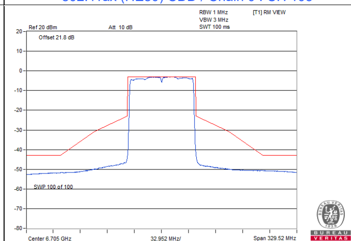
802.11ax (HE80) CDD / Chain 0 : CH 151
