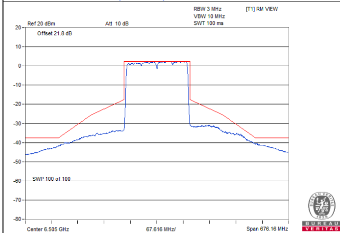
802.11ax (HE160) CDD / Chain 1 : CH 111
