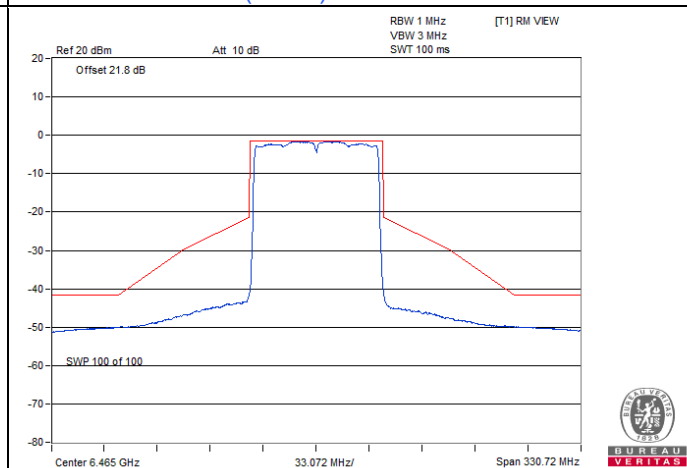
802.11ax (HE80) CDD / Chain 0 : CH 103
