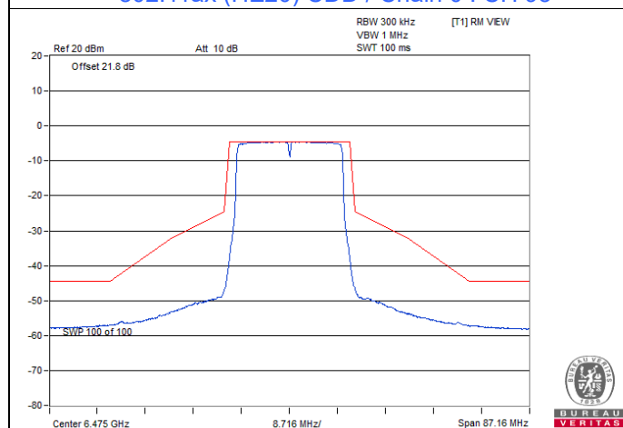
802.11ax (HE20) CDD / Chain 0 : CH 105
