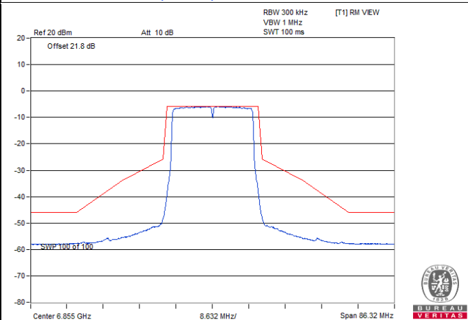
802.11ax (HE20) CDD / Chain 1 : CH 181
