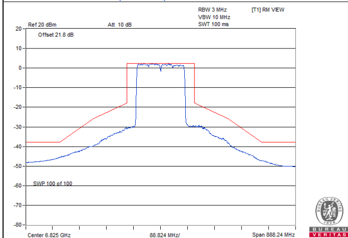
802.11ax (HE160) CDD / Chain 1 : CH 175
