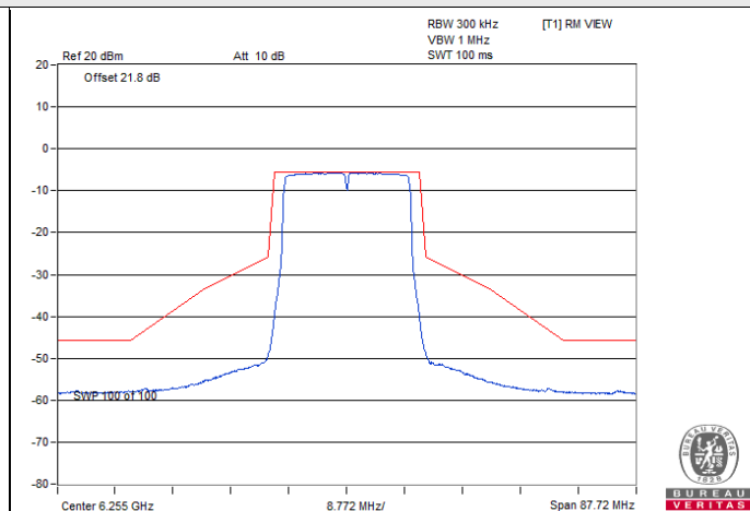
802.11ax (HE20) CDD / Chain 0 : CH 61
