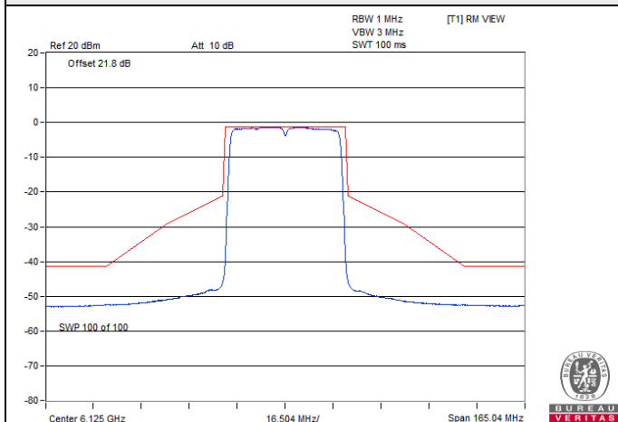
802.11ax (HE40) CDD / Chain 1 : CH 35
