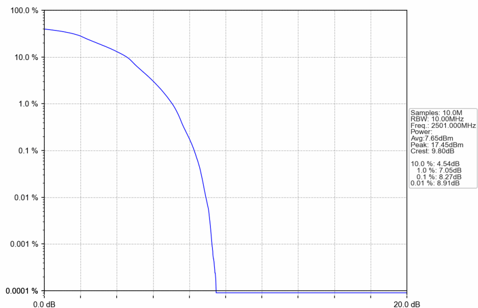
Band41_10MHz_16QAM_LCH_2501MHz_RB_27_0_NTNV
