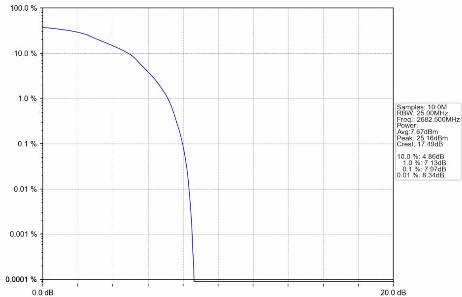
Band41_15MHz_16QAM_HCH_2682.5MHz_RB_27_48_NTNV
