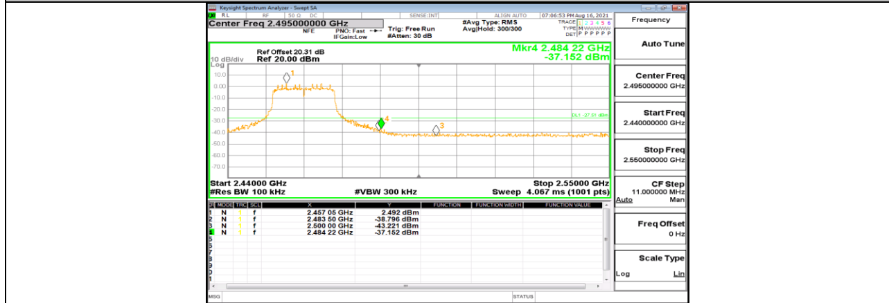
11N20MIMO_Ant1_High_2462
