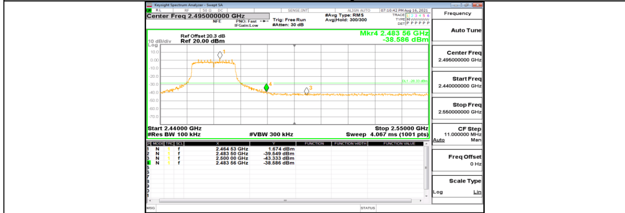
11N20MIMO_Ant2_High_2462
