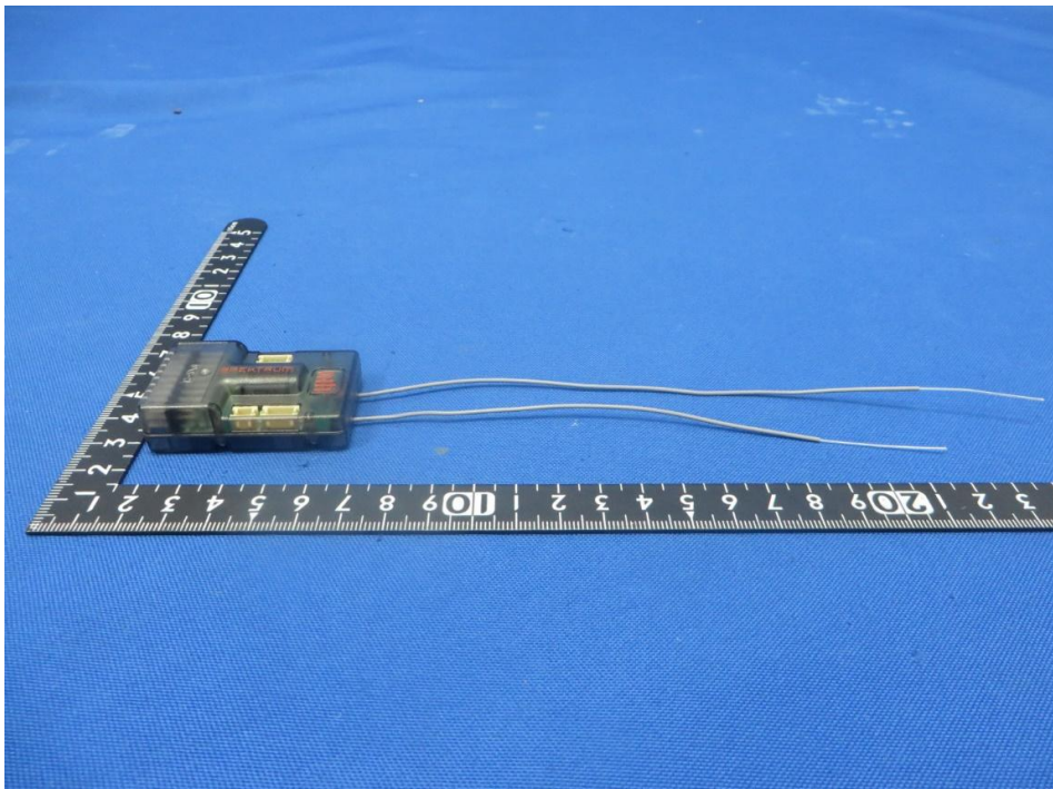
(2) EUT Photo
