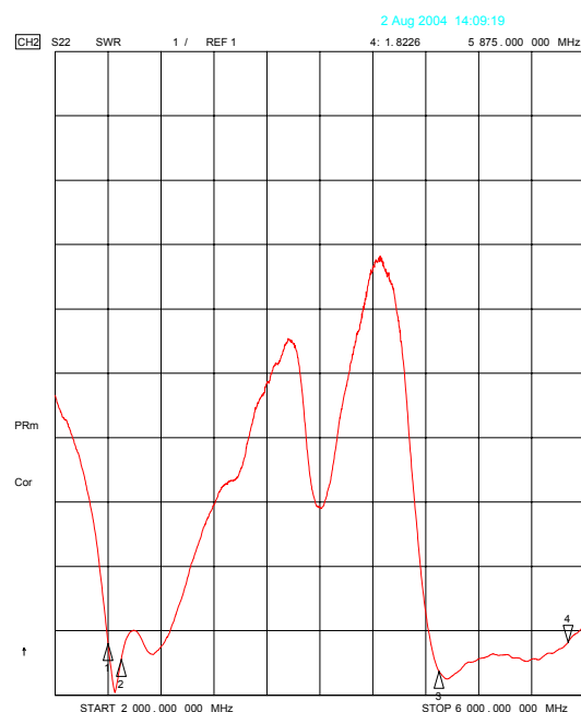
VSWR
