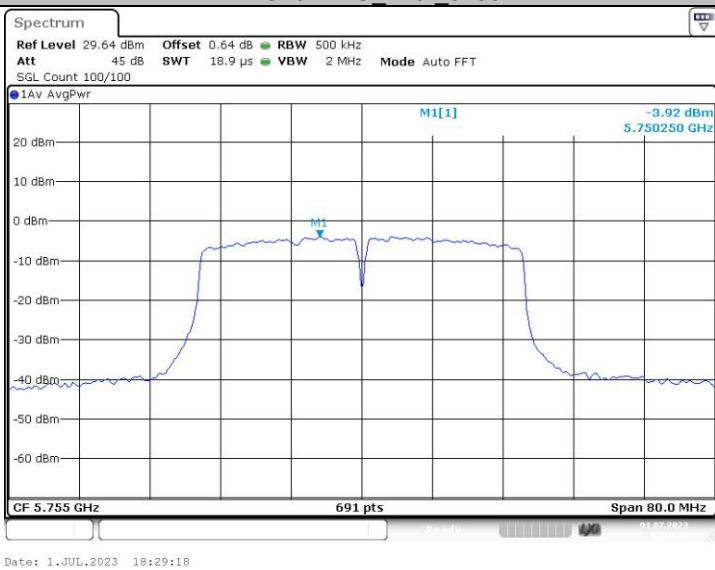
11AC40MIMO_Ant2_5755
