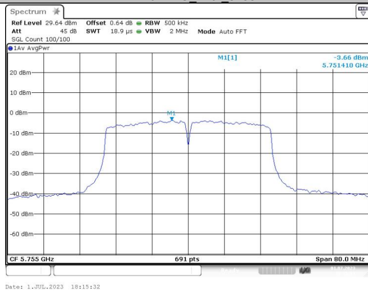
11N40MIMO_Ant2_5755
