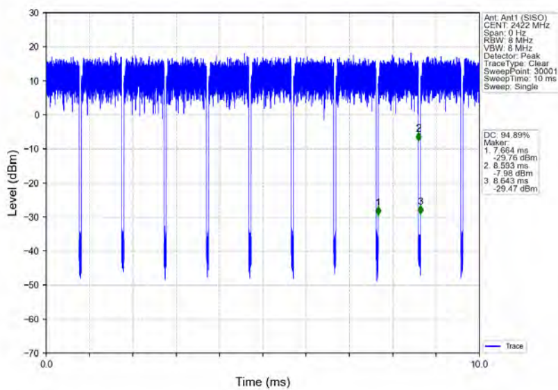
802.11n(HT40)_LCH_2422MHz_Ant1 (SISO)_NTNV
