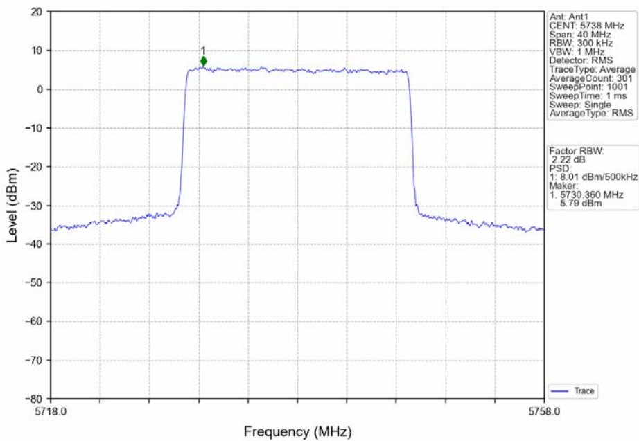
16QAM 20MHz_LCH_5738MHz_Ant1_NTNV
