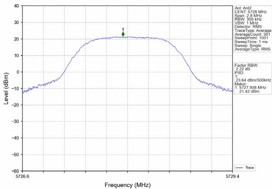
QPSK 1.4MHz_LCH_5728MHz_Ant2_NTNV
