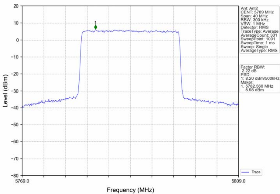
16QAM 20MHz_MCH_5789MHz_Ant2_NTNV
