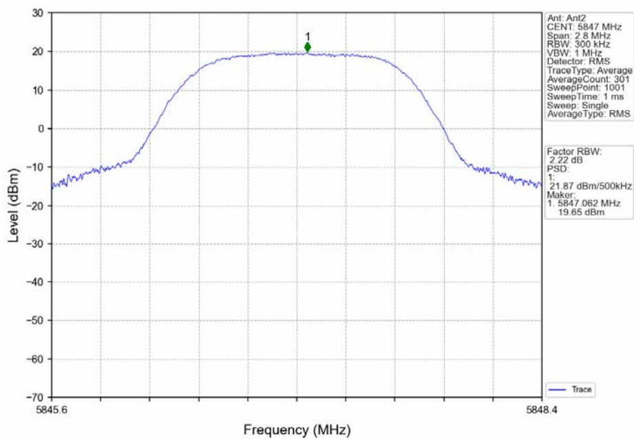
16QAM 1.4MHz_HCH_5847MHz_MIMO_NTNV
