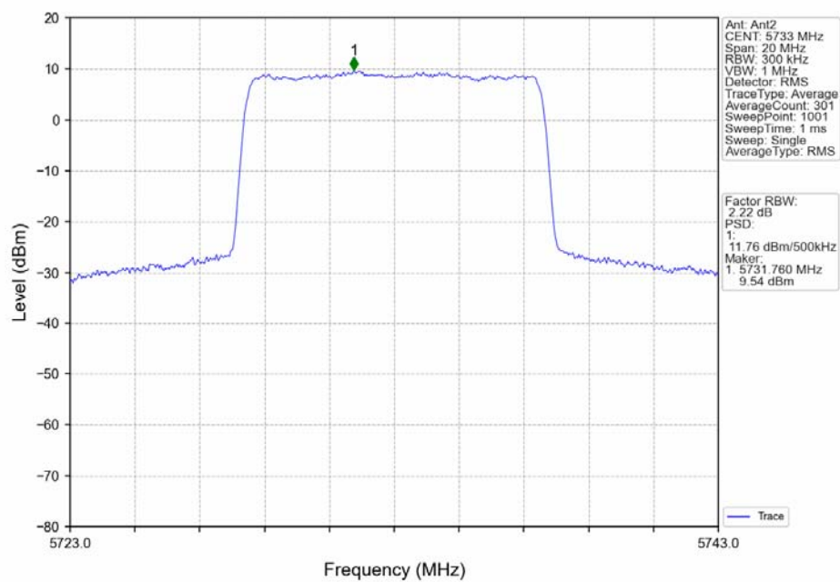
QPSK 10MHz_LCH_5733MHz_Ant2_NTNV
