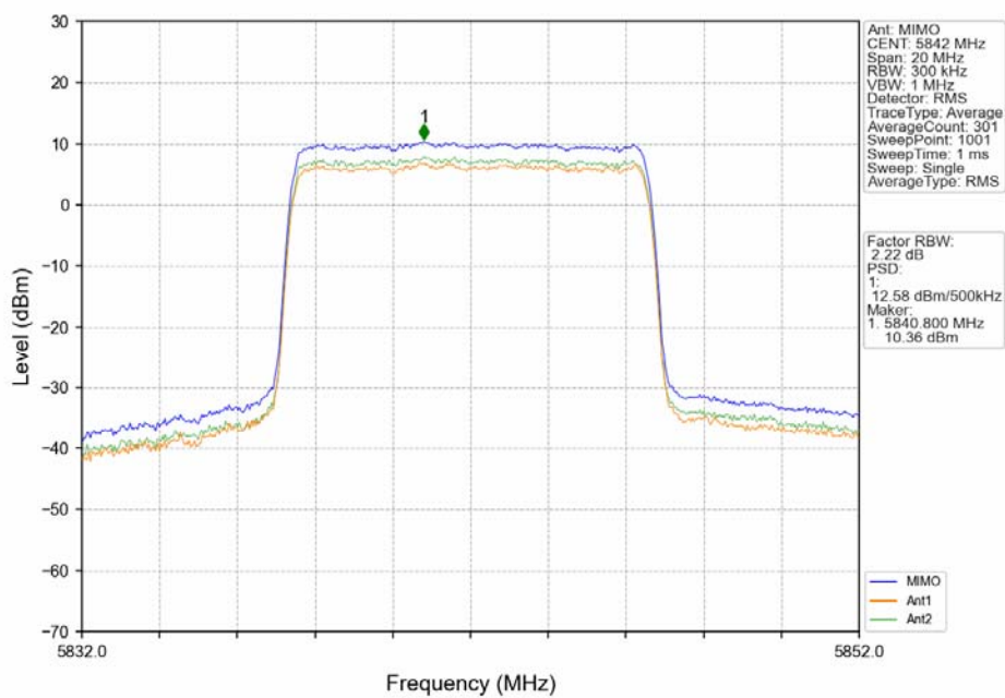
16QAM 10MHz_HCH_5842MHz_MIMO_NTNV
