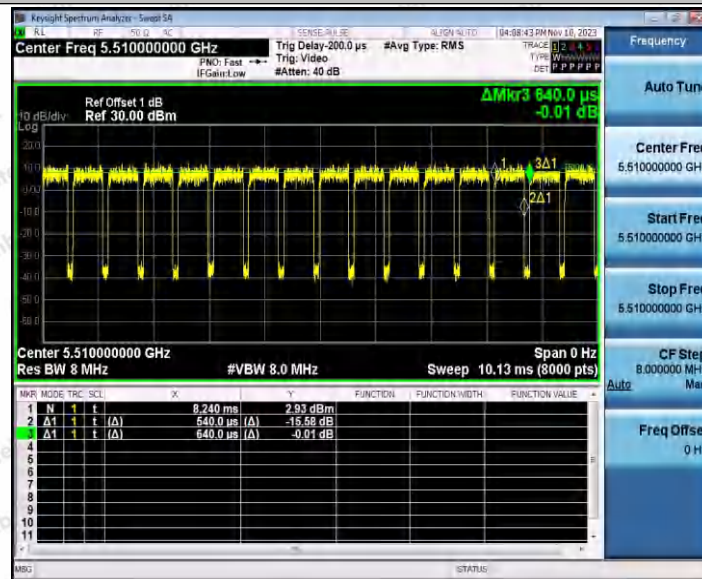
11AX40SISO_Ant2_5510
