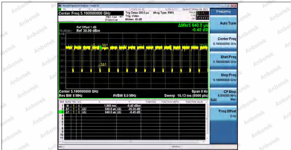
11AX40ISO_Ant2_5190
