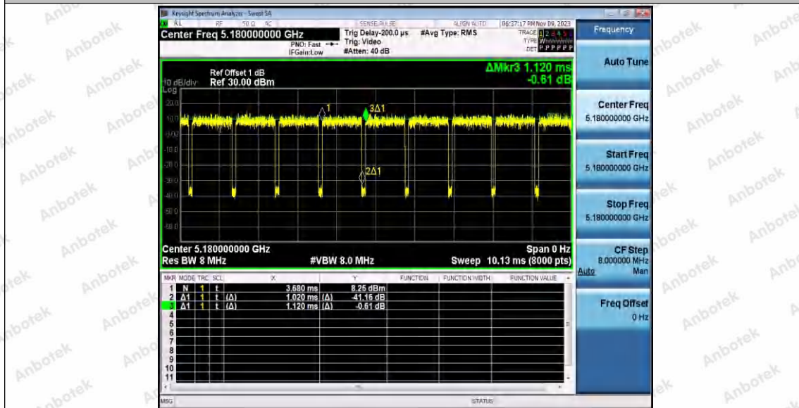
11AX20SISO_Ant2_5180
