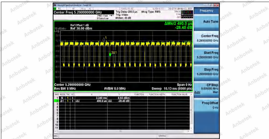
11AX80ISO_Ant2_5290
