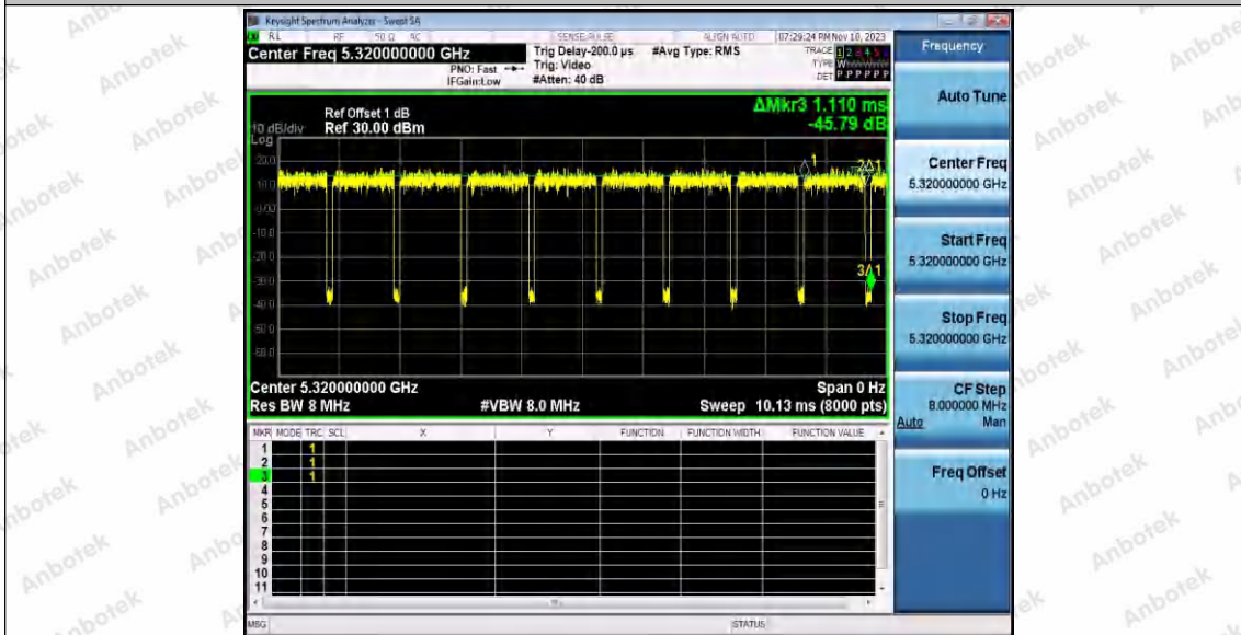
11AX20SISO_Ant2_5320
