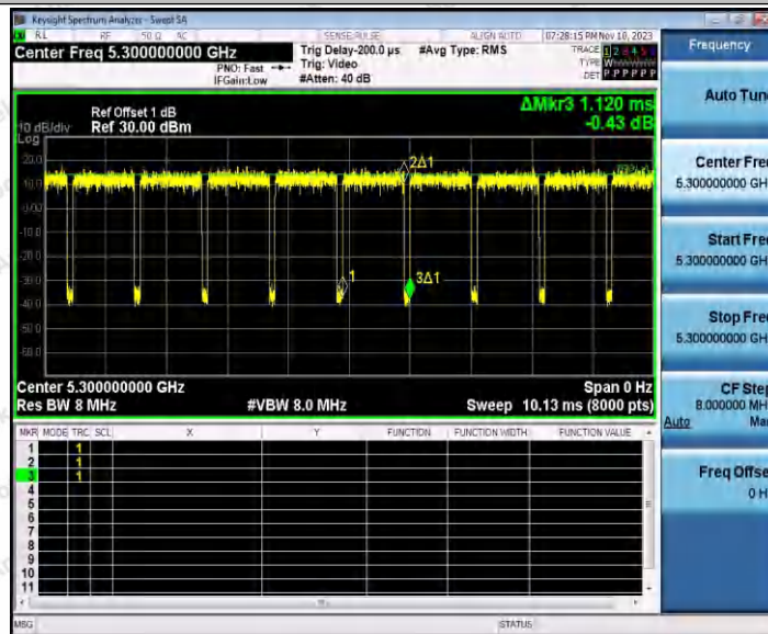
11AX20SISO_Ant2_5300
