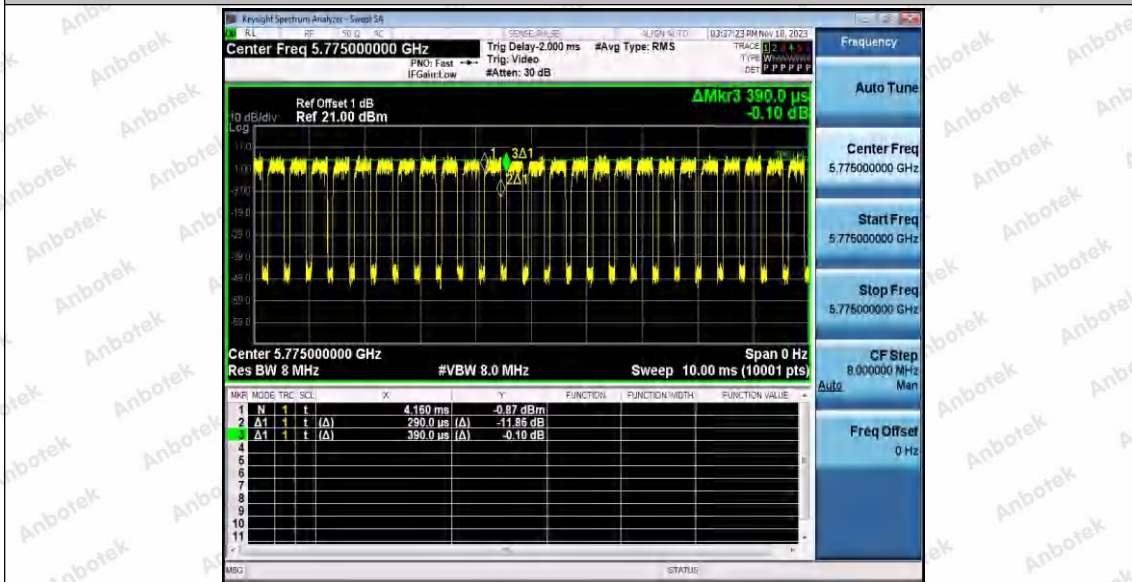
11AX80ISO_Ant2_5775
