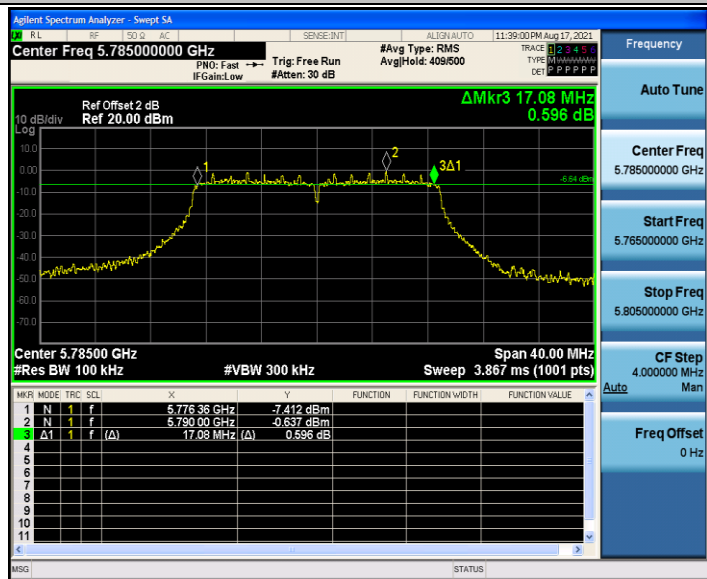
11AC20MIMO_Ant2_5785
