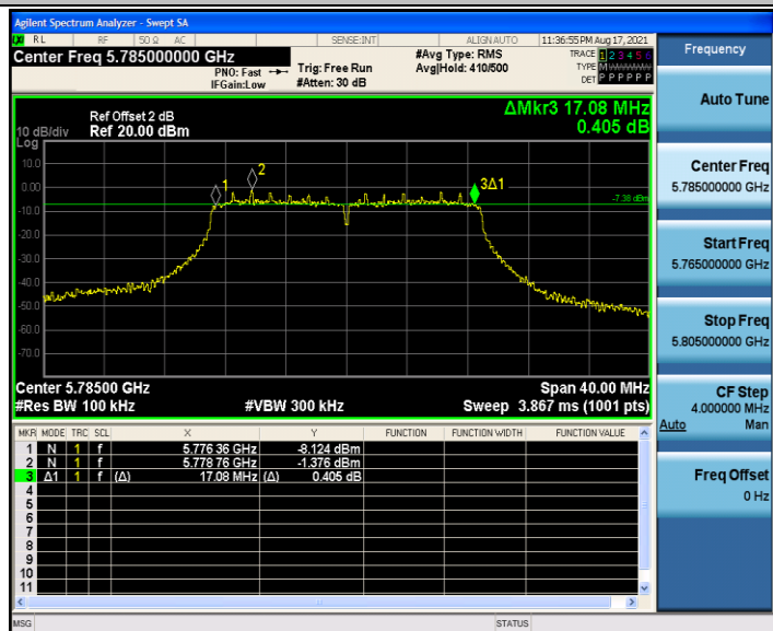
11AC20MIMO_Ant2_5785
