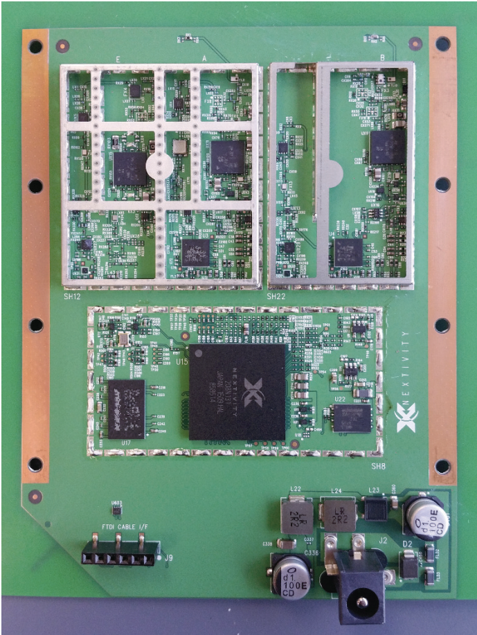
PCB Side_2_no shield – NU
