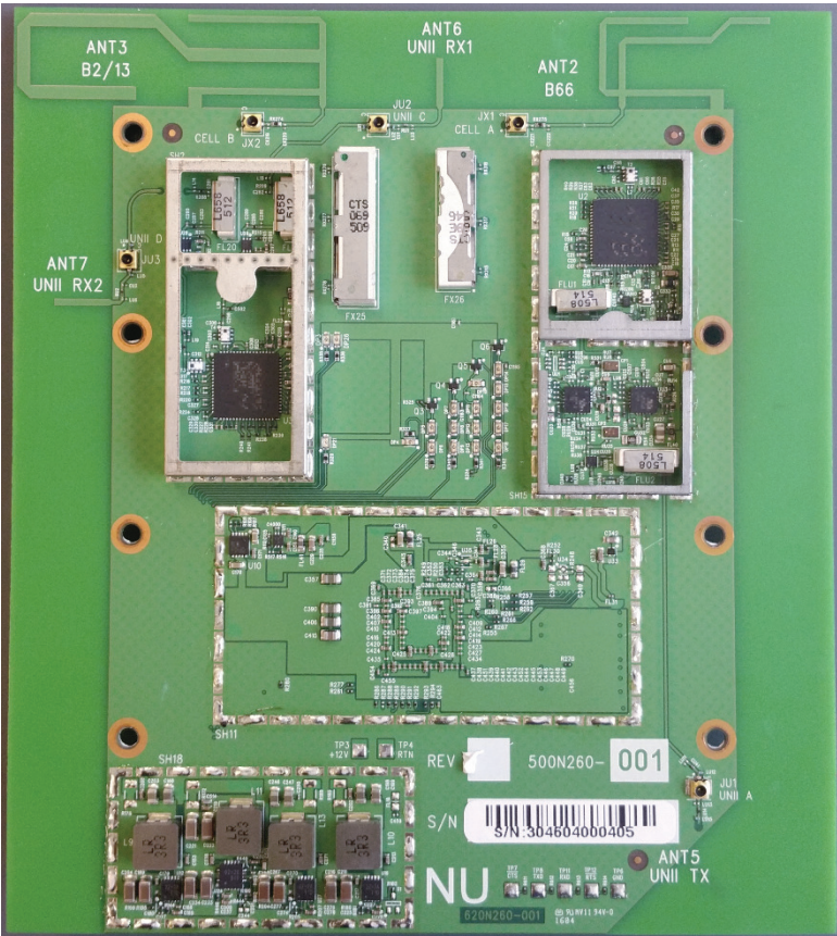
PCB Side_1_no shield – NU
