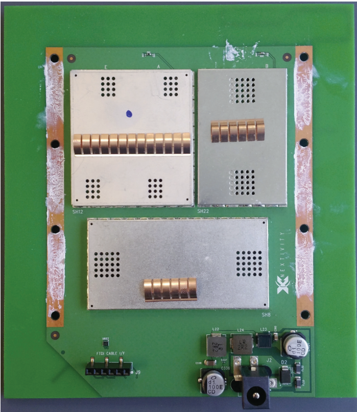
PCB Side_2 – NU
