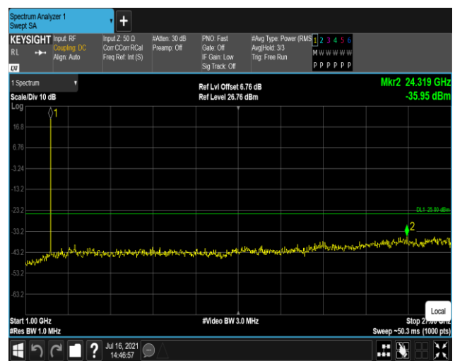
Band7-5MHz-QPSK-21425:1000~27000MHz
