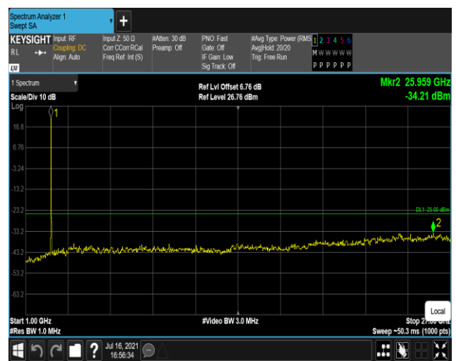
Band38-20MHz-QPSK-38000:1000~27000MHz
