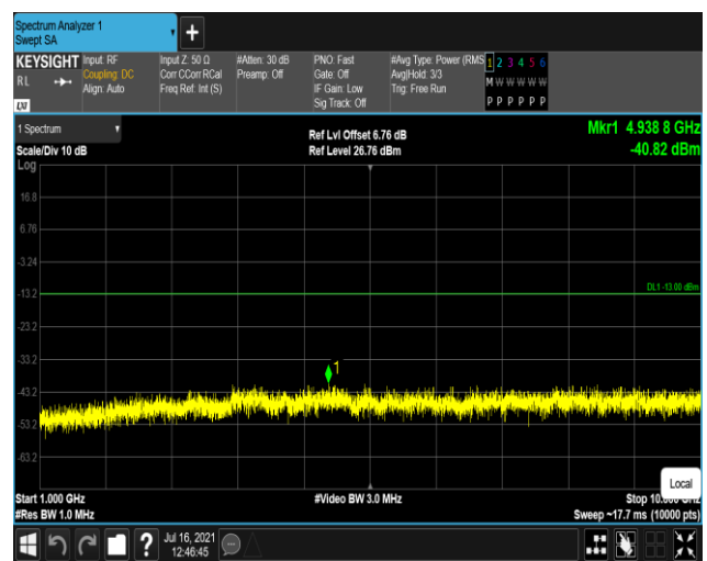
Band5-10MHz-QPSK-20525:1000~10000MHz
